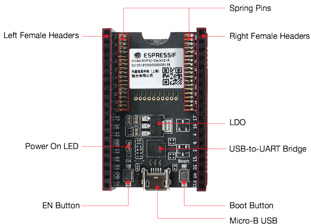
图 2: ESP32-DevKitS-R - 正面
