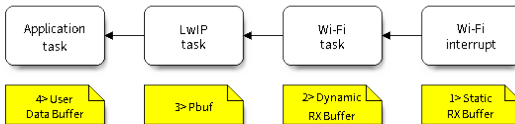
图 85: 接收数据缓冲区分配
