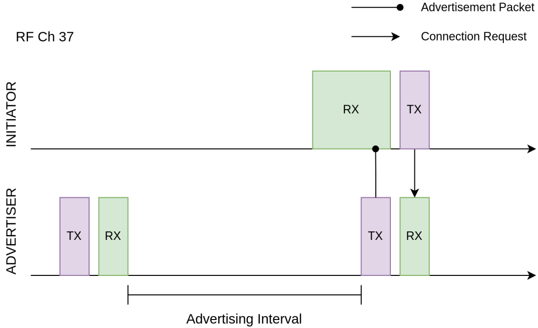
图 20: 连接的发起
