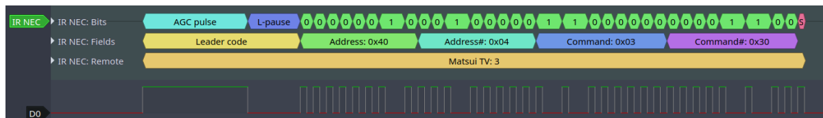
图 20: 红外 NEC 帧
