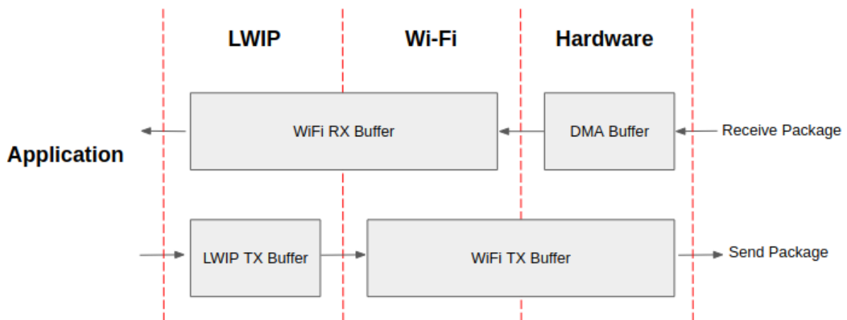
图 83: ESP32 数据路径
