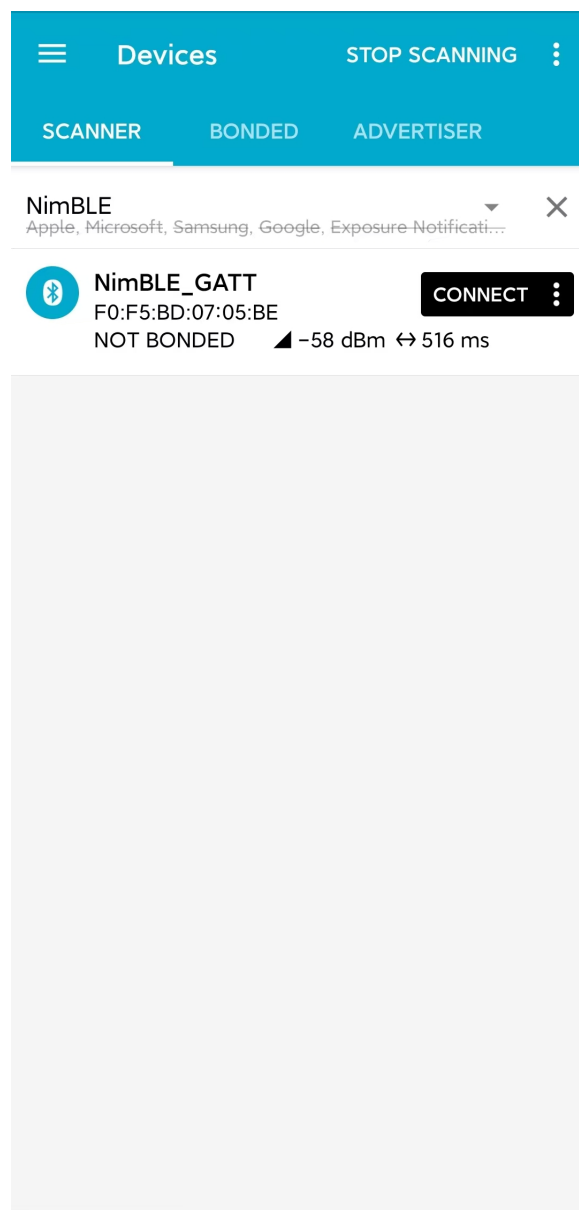
图 7: 扫描设备
