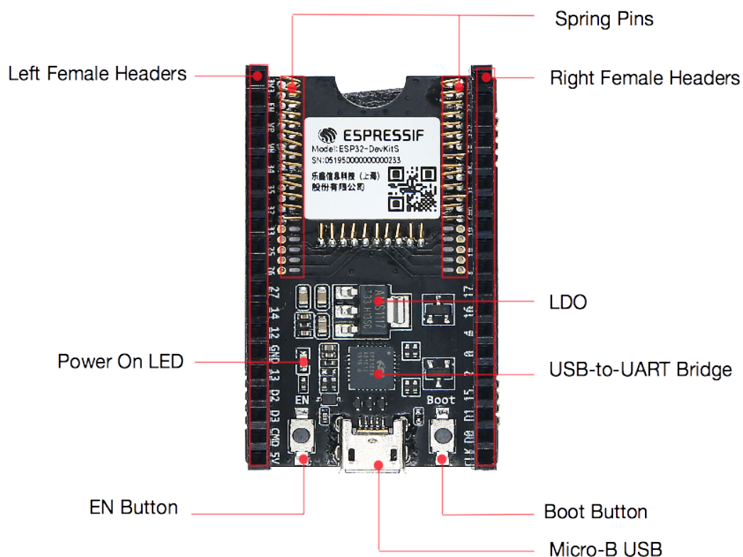
图 1: ESP32-DevKitS - 正面
