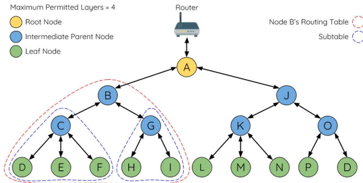
图 47: ESP-WIFI-MESH 路由表示例
