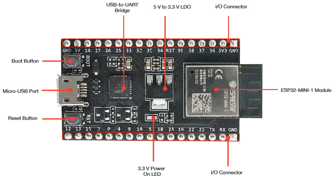
图 6: ESP32-DevKitM-1 - 正面
