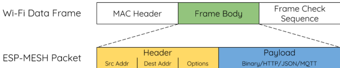
图 54: ESP-WIFI-MESH 数据包
