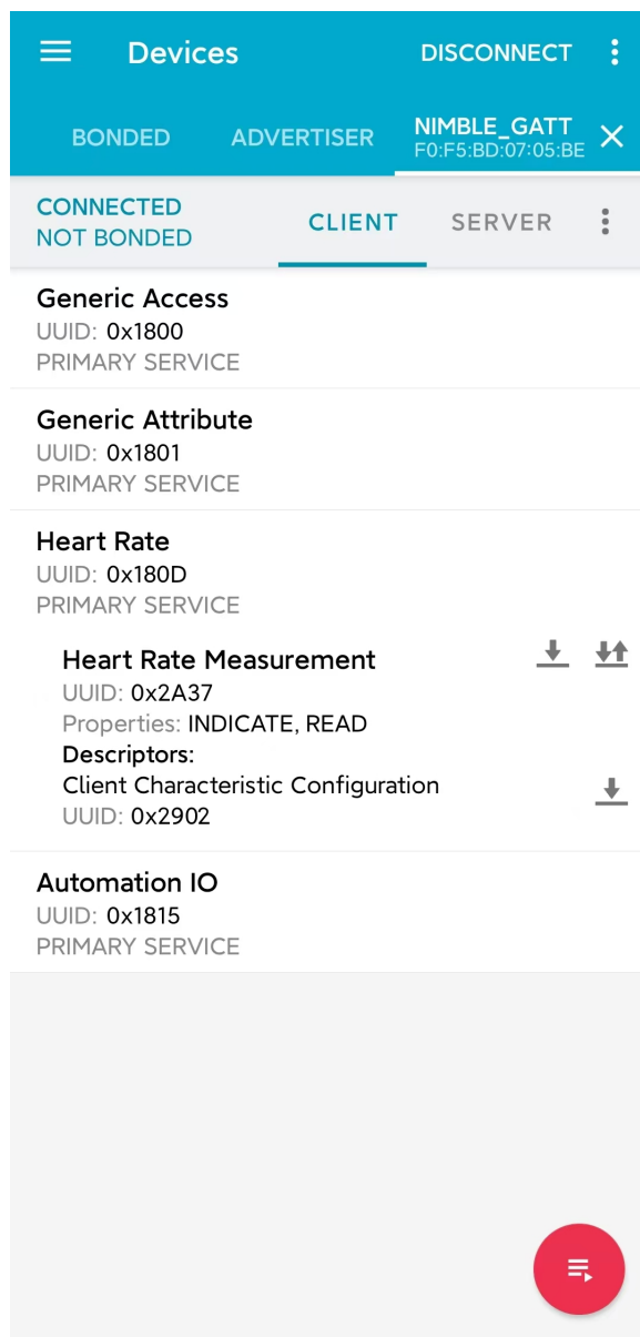
图 12: Heart Rate Service
