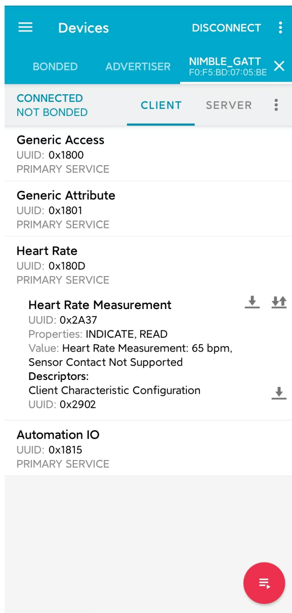
图 13: 对心率特征数据进行读访问
