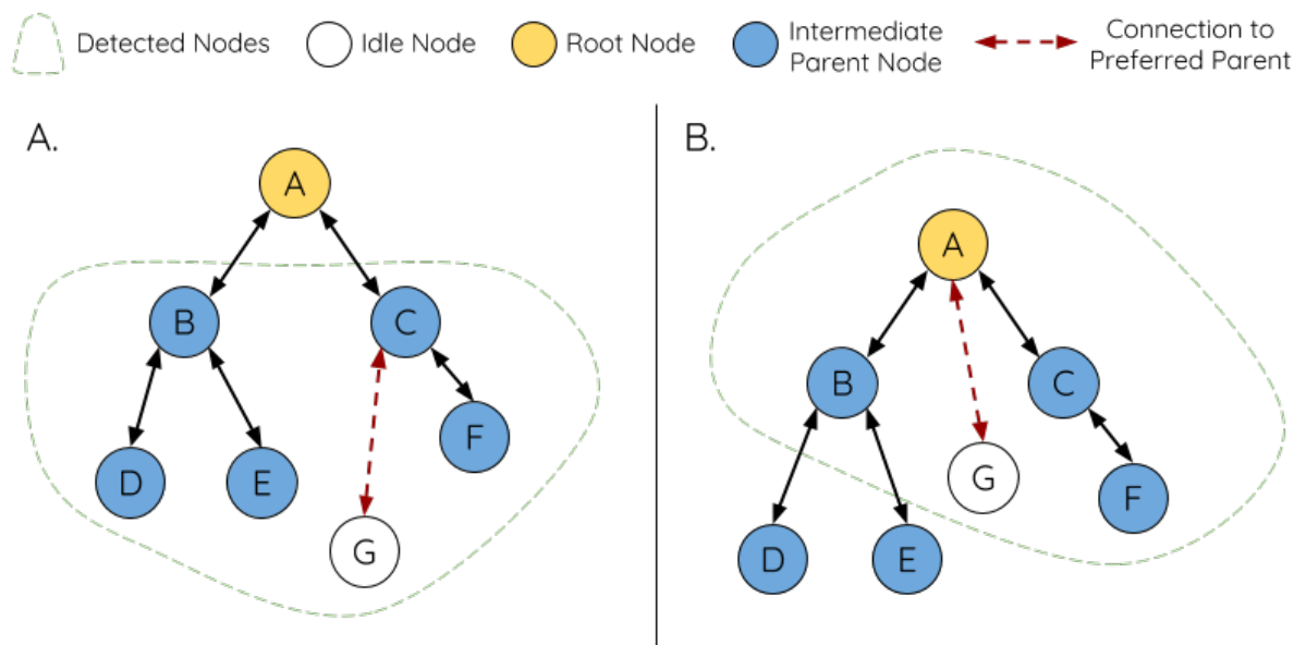
图 46: 首选父节点选择
