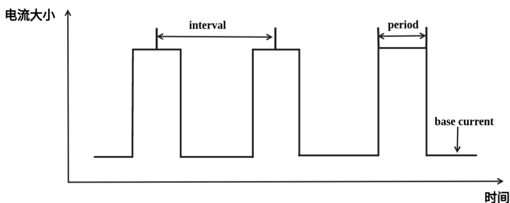
图 55: 理想情况下 Wi-Fi 场景低功耗模式电流图
