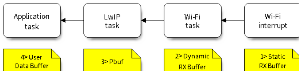
图 35: 接收数据缓冲区分配
