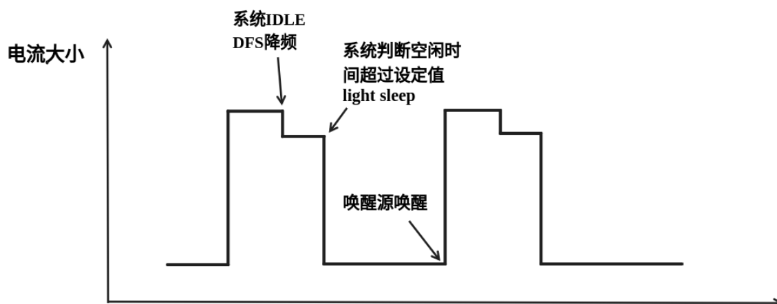
图 50: Auto Light-sleep 模式理想电流图
