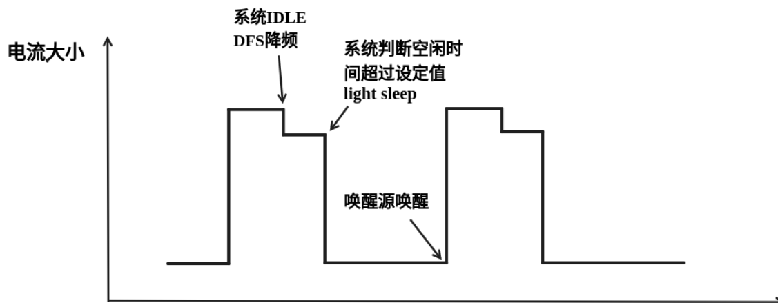
图 50: Auto Light-sleep 模式理想电流图
