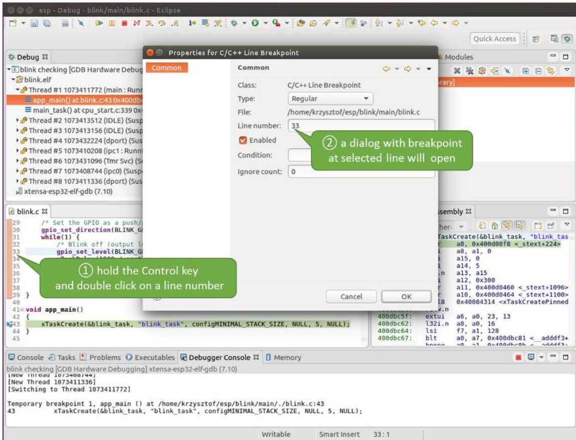
图 37: 设置断点
