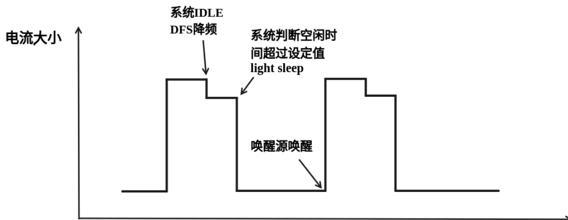
图 71: Auto Light-sleep 模式理想电流图
