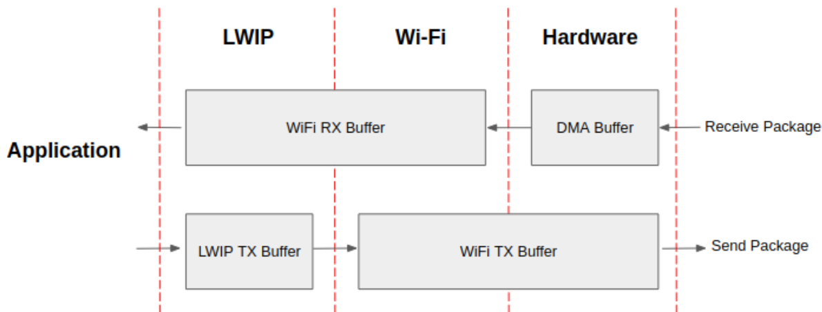
图 61: ESP32-C3 数据路径
