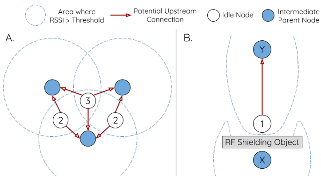
图 24: RSSI 閾值的影响
