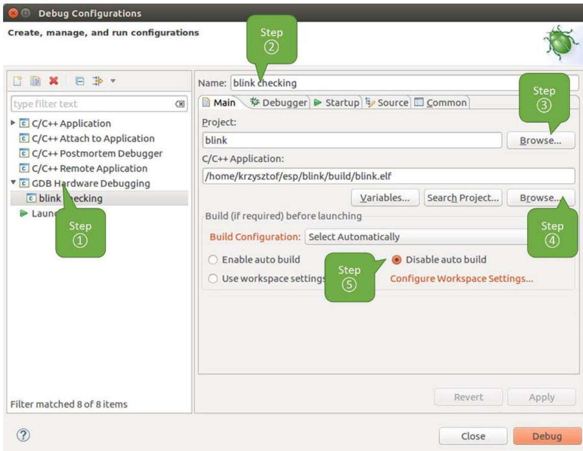
图 57: GDB 硬件调试的配置 - Main 选项卡
