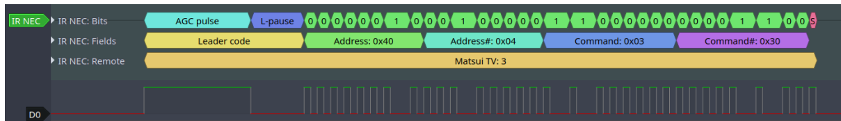
图 18: 红外 NEC 帧
