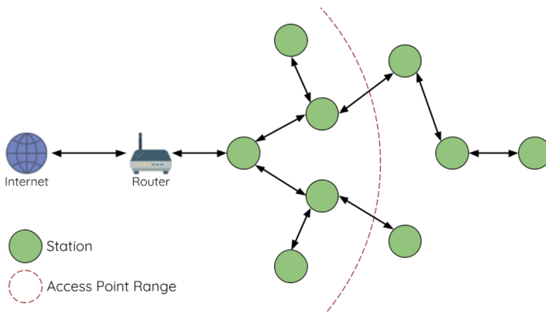
图 21: ESP-WIFI-MESH 网络架构示意图
