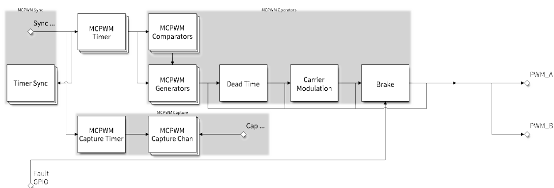
图 10: MCPWM Overview
