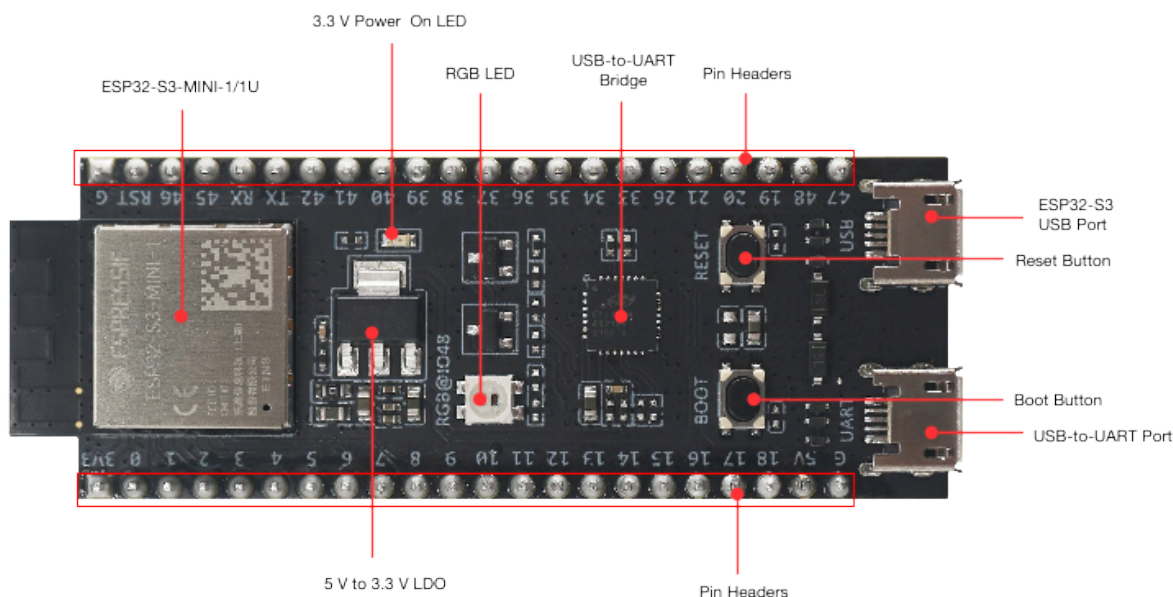
图 10: ESP32-S3-DevKitM-1 - 正面
