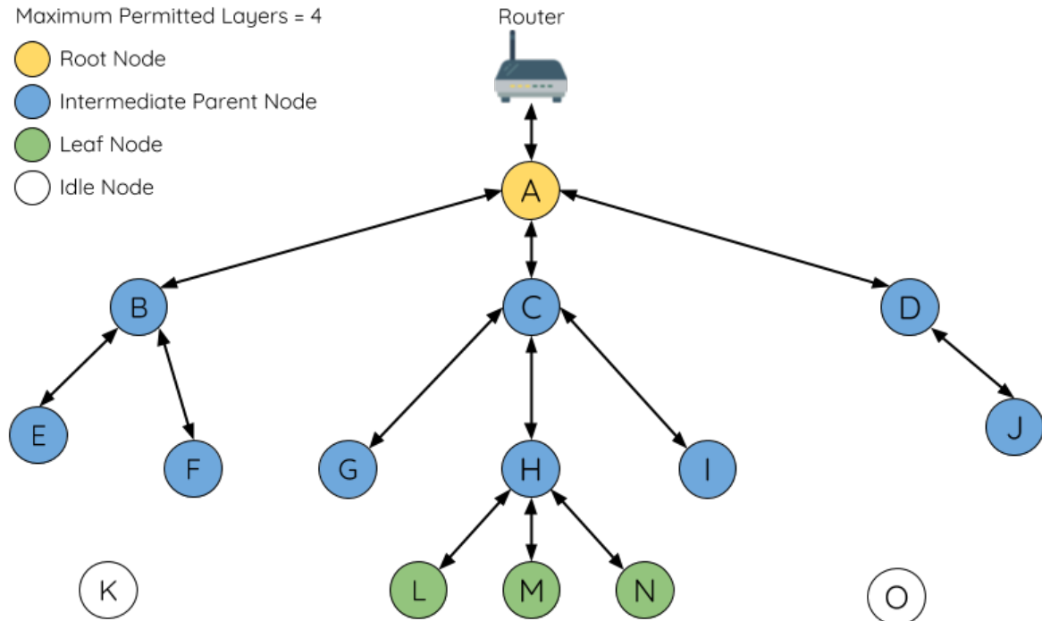
图 23: ESP-WIFI-MESH 节点类型
