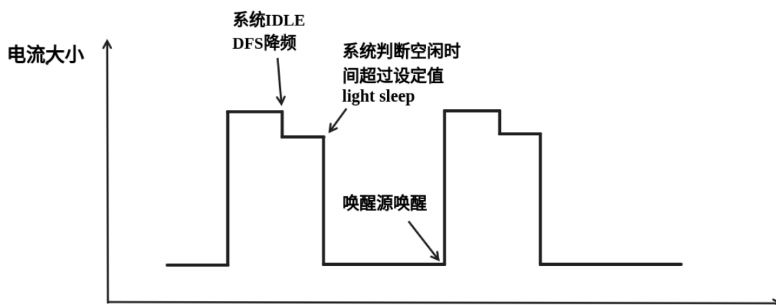
图 78: Auto Light-sleep 模式理想电流图
