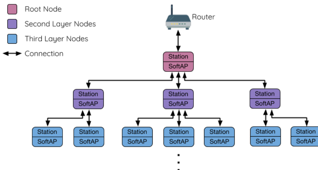
图 22: ESP-WIFI-MESH 树型拓扑
