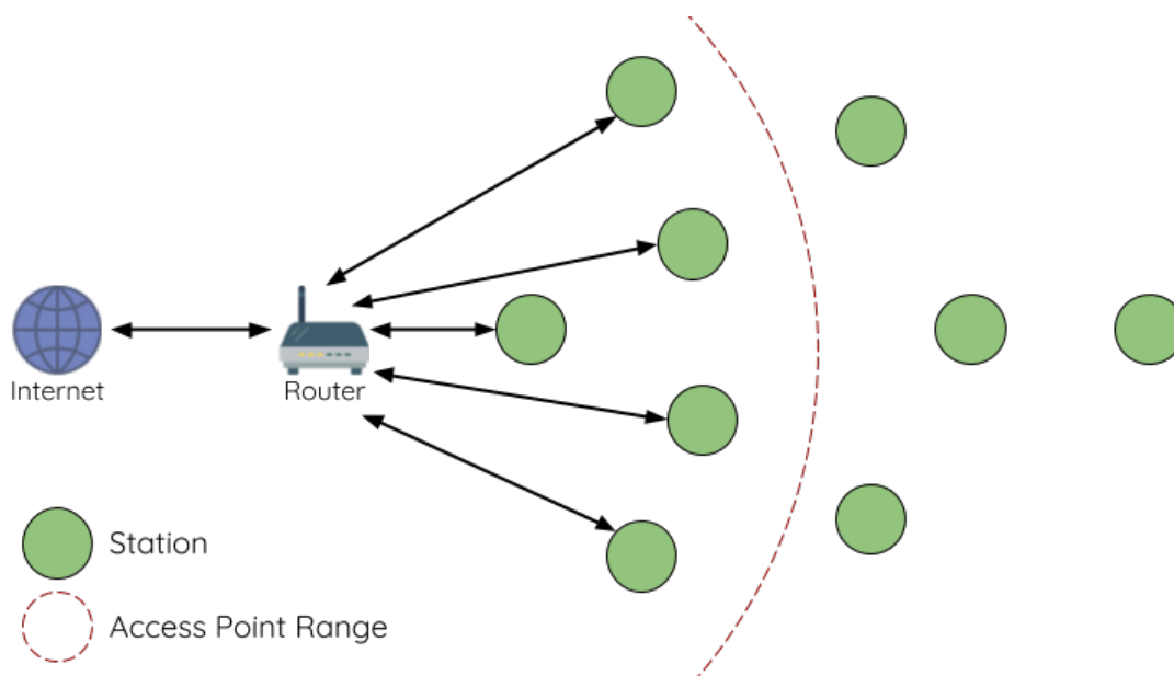
图 20: 传统 Wi-Fi 网络架构
