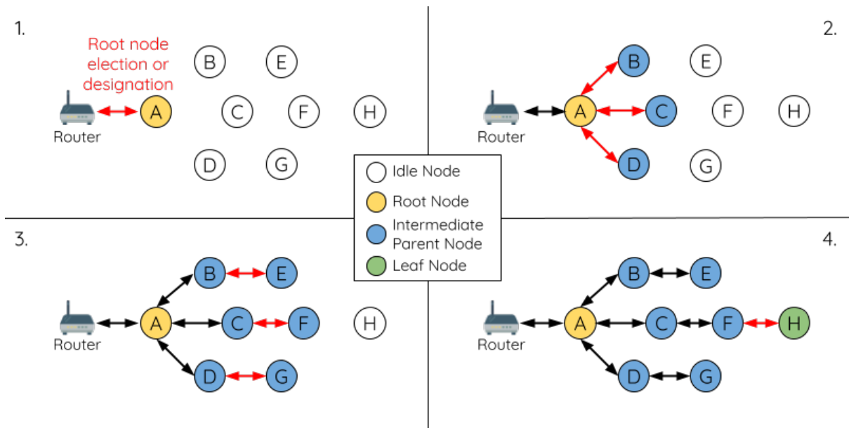
图 27: ESP-WIFI-MESH 网络构建过程
