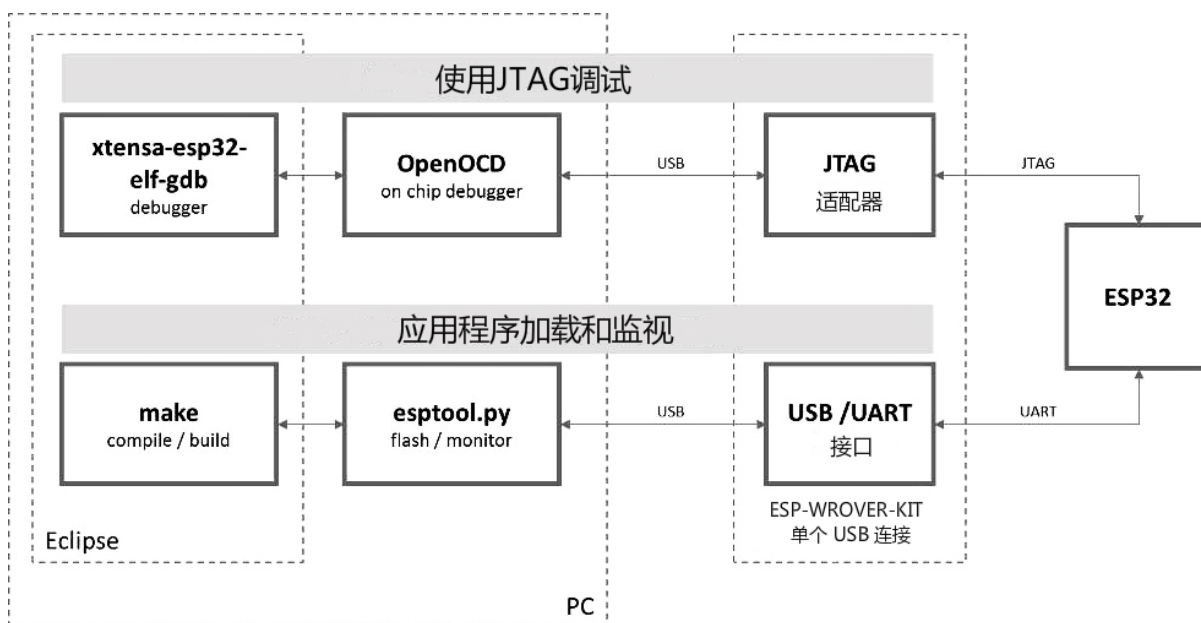
图 56: JTAG 调试 - 概述图
