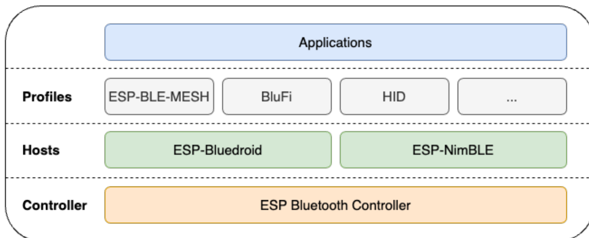
图 2: ESP32-S3 蓝牙协议栈架构
