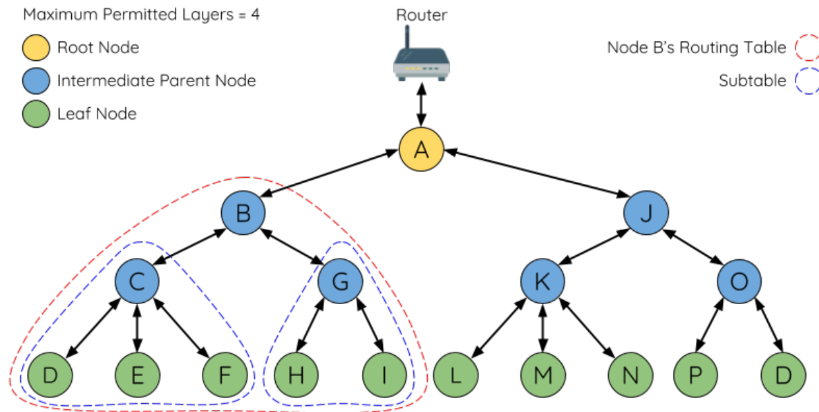
图 46: ESP-WIFI-MESH 路由表示例
