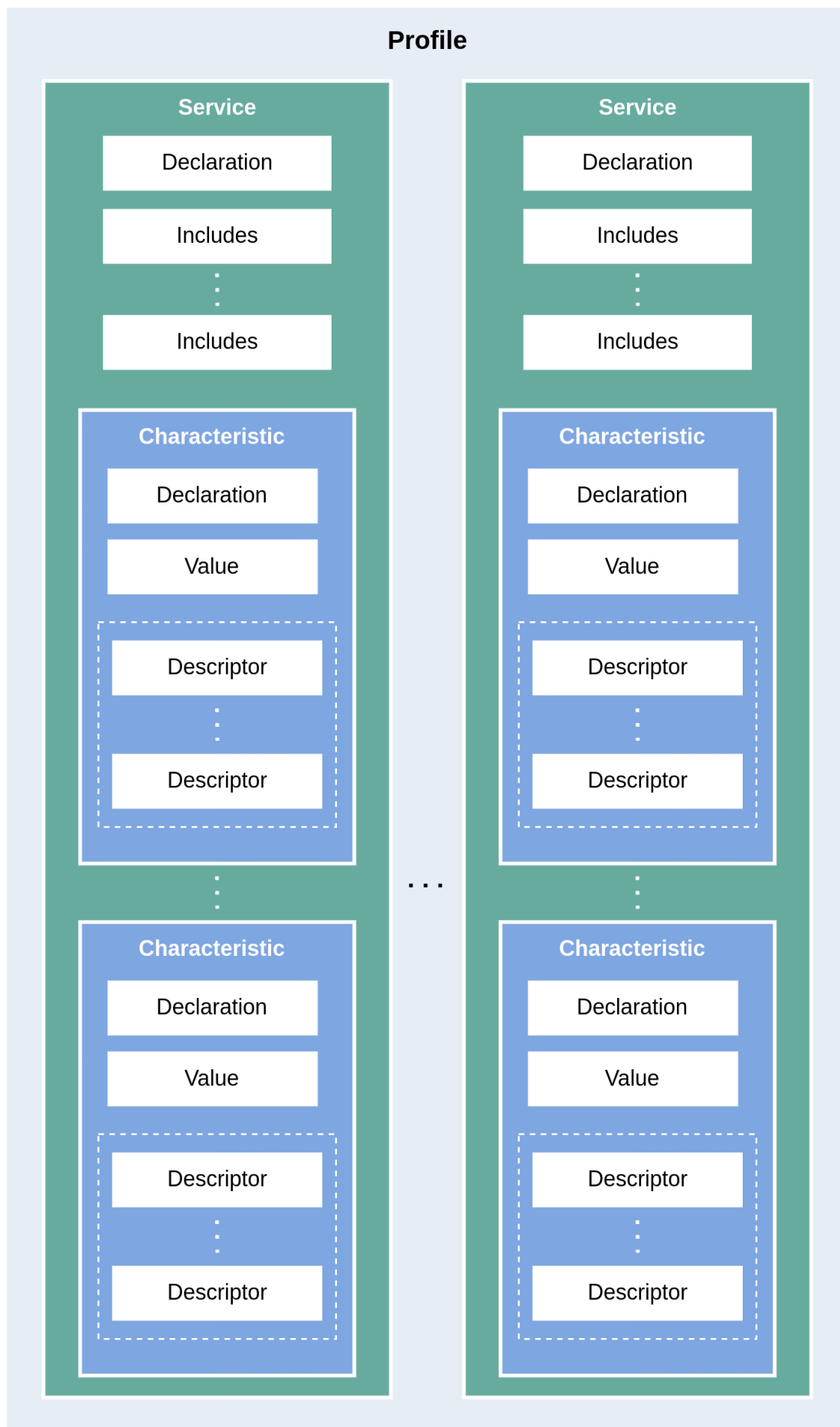
图 5: GATT 中的层次关系
