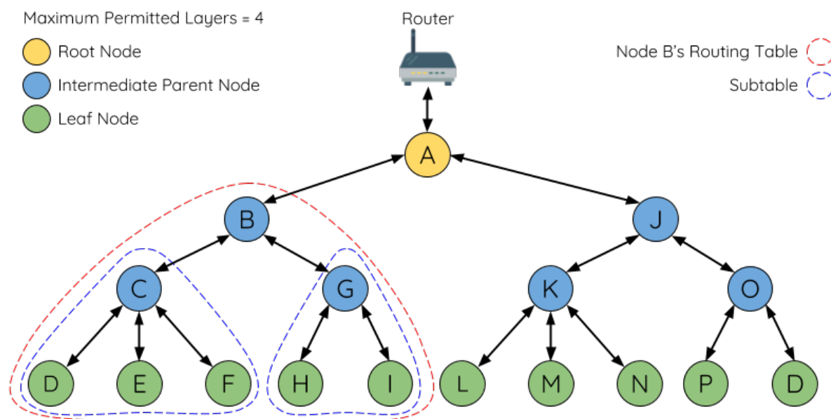
图 29: ESP-WIFI-MESH 路由表示例
