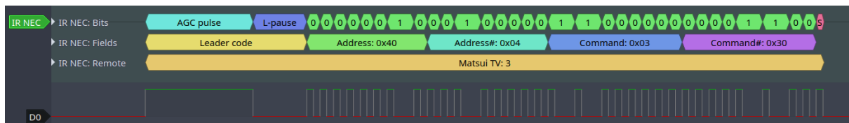
图 21: 红外 NEC 帧
