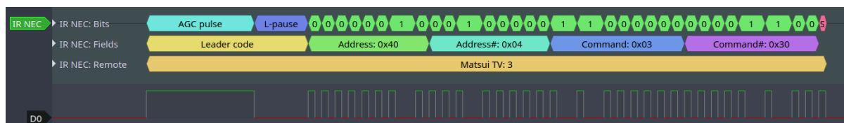
图 21: 红外 NEC 帧
