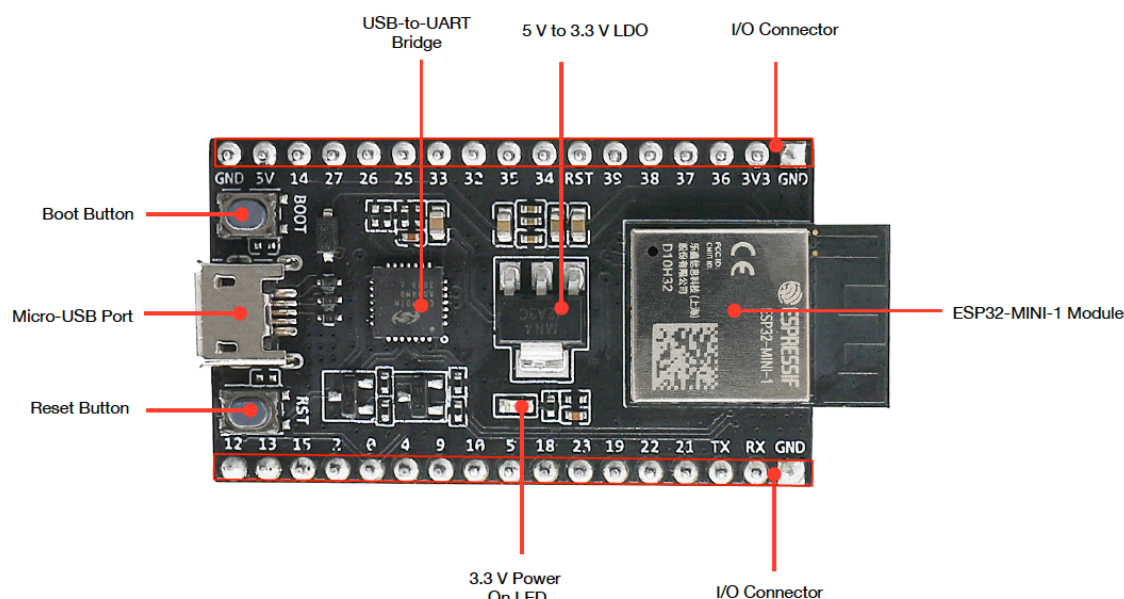
图 6: ESP32-DevKitM-1 - 正面
