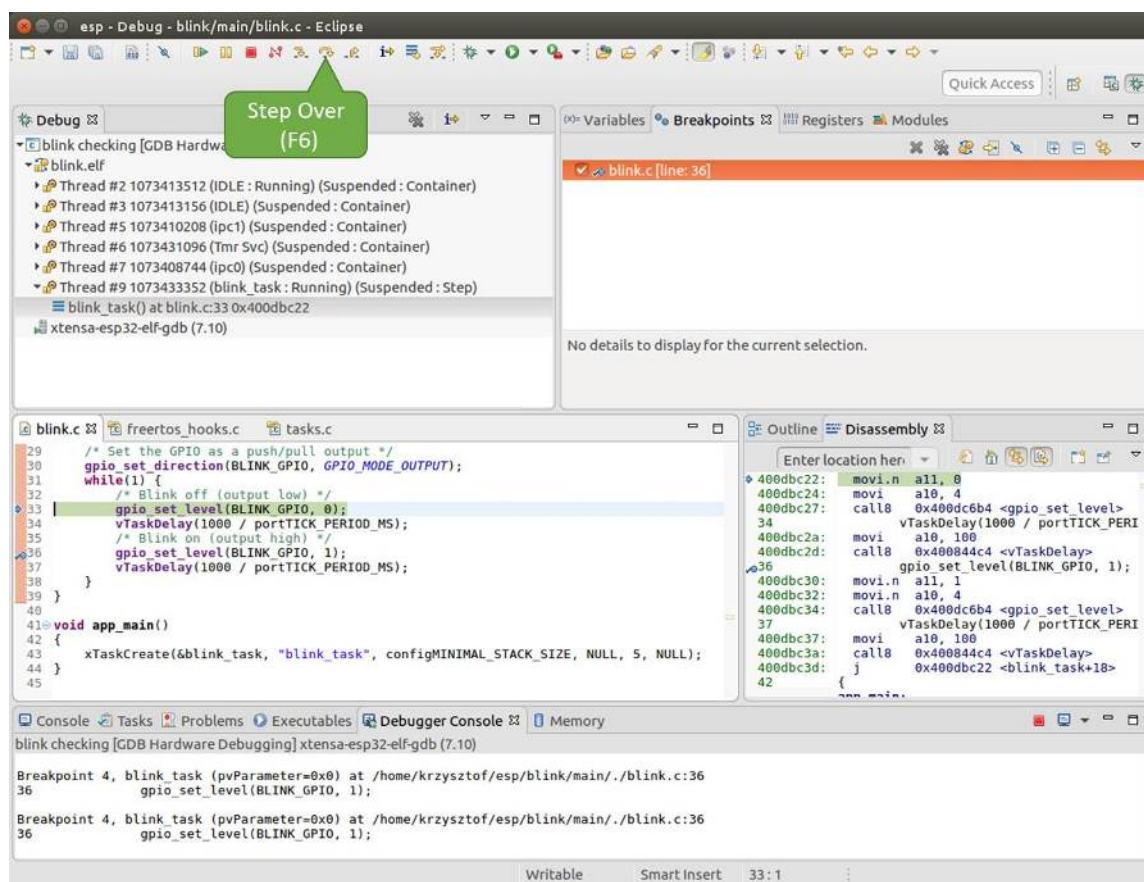
图 71: 使用“Step Over (F6)”单步执行代码
