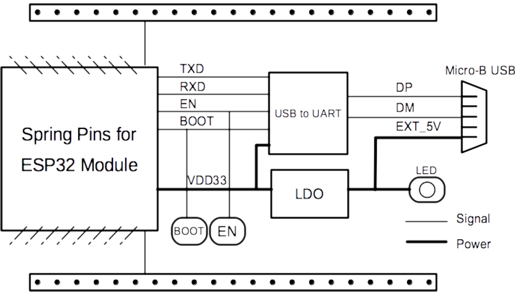
图 5: ESP32-DevKitS(-R) (点击放大)
