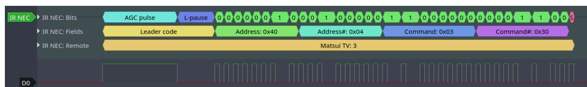
图 21: 红外 NEC 帧
