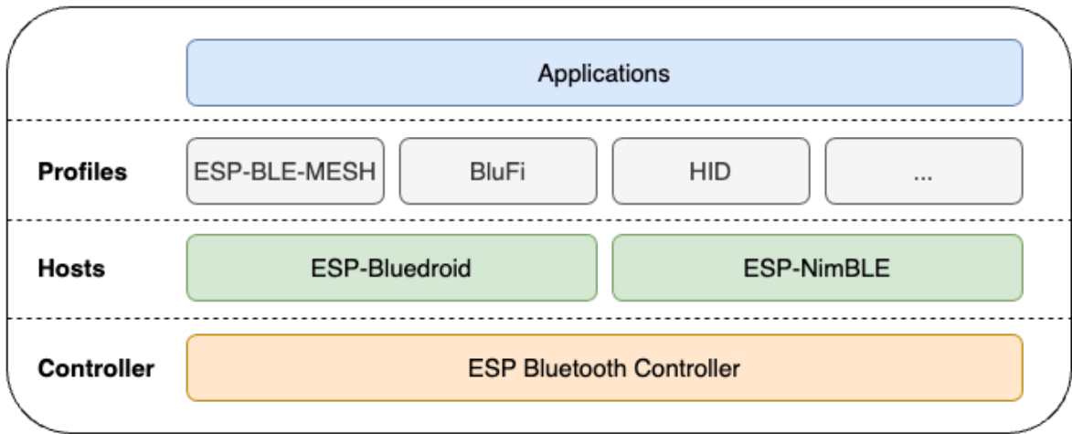
图 3: ESP32 蓝牙协议栈架构
