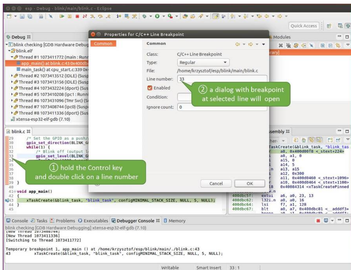
图 68: 设置断点
