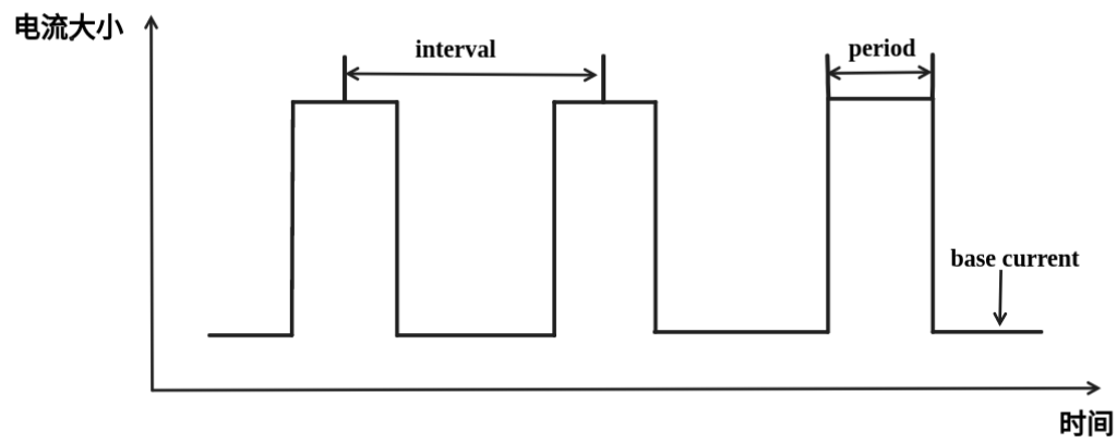
图 105: 理想情况下 Wi-Fi 场景低功耗模式电流图
