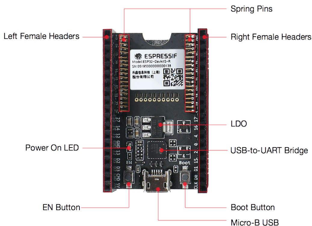
图 2: ESP32-DevKitS-R - 正面
