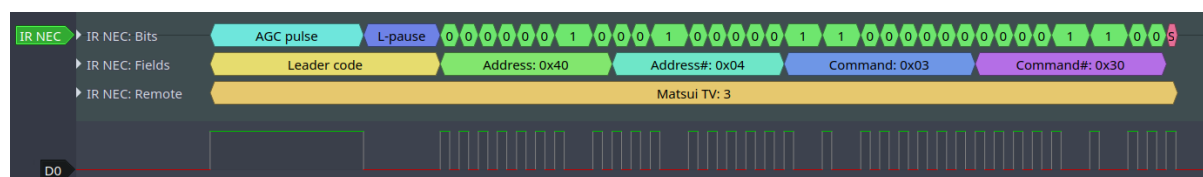
图 21: 红外 NEC 帧
