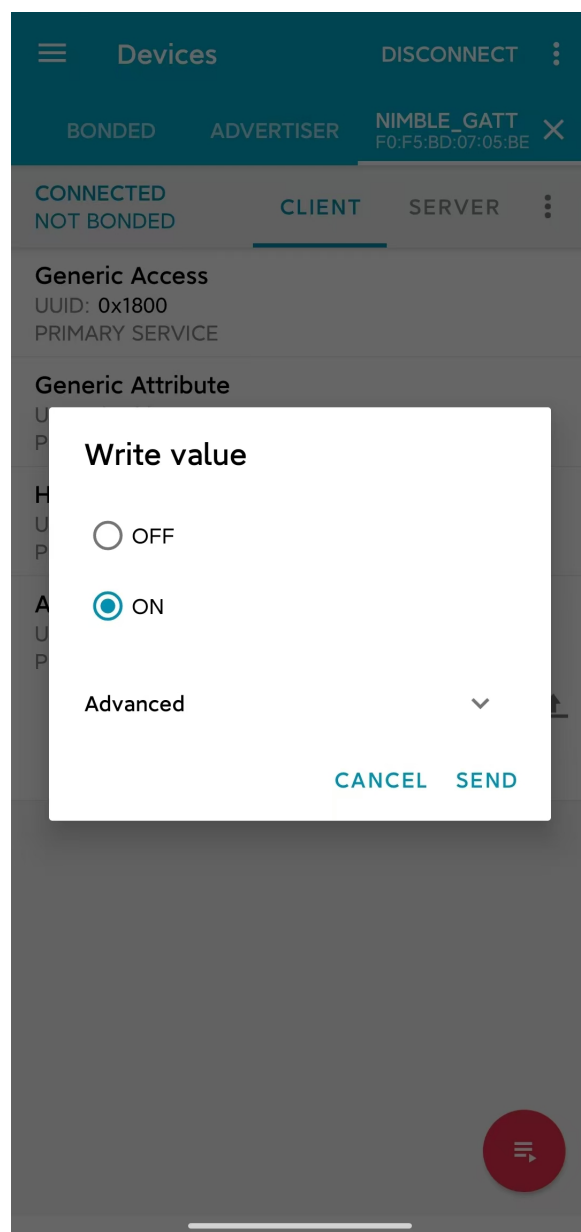
图 11: 对 LED 特征数据进行写访问
