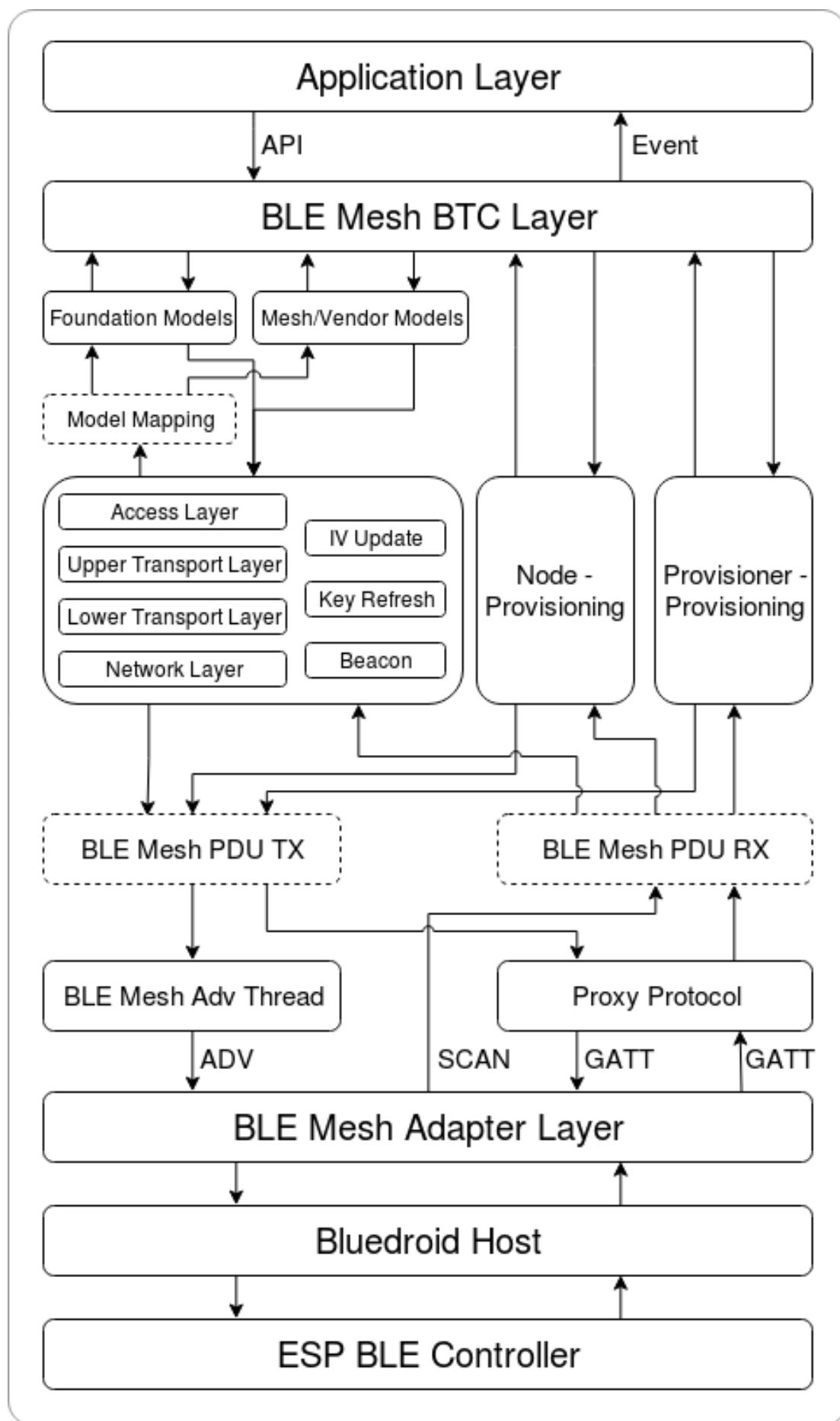
图 35: 图 2.1 ESP-BLE-MESH 架构实现图
