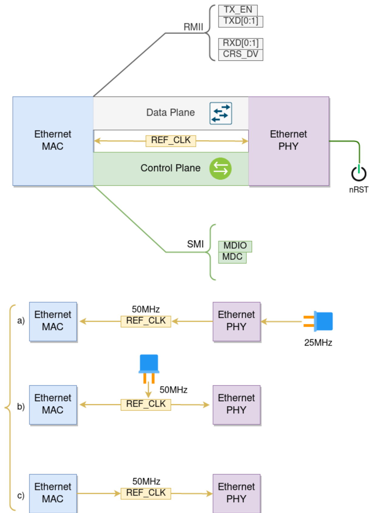
图 5: 以太网 RMI 接口
