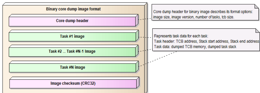
图 41: 核心转储二进制镜像文件格式
