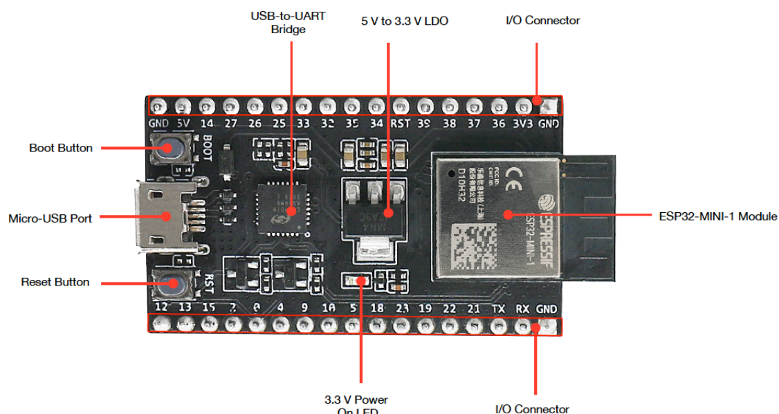
图 6: ESP32-DevKitM-1 - 正面
