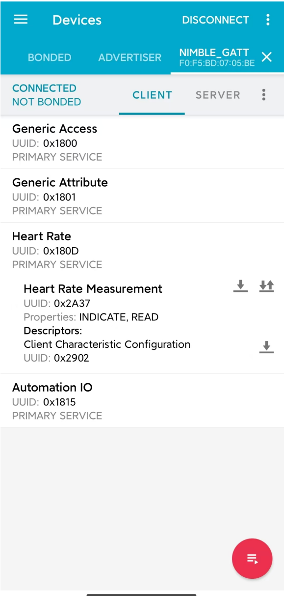
图 12: Heart Rate Service
