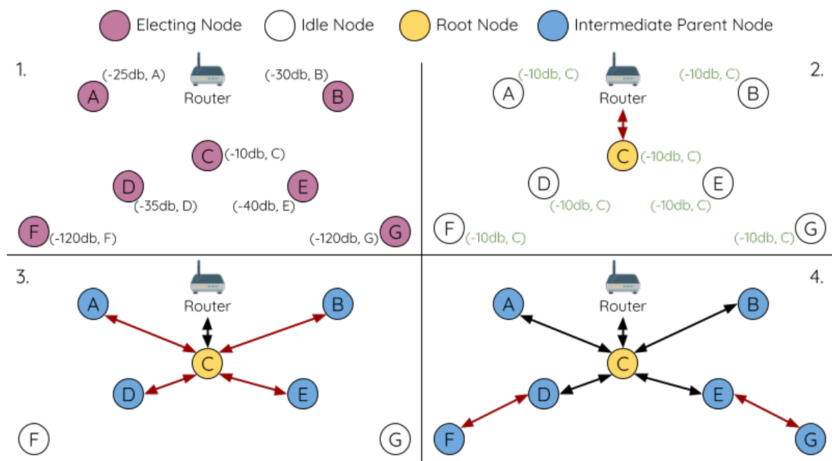
图 51: 根节点选举示例
