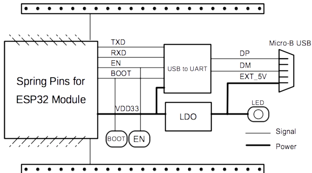
图 5: ESP32-DevKitS(-R) (点击放大)
