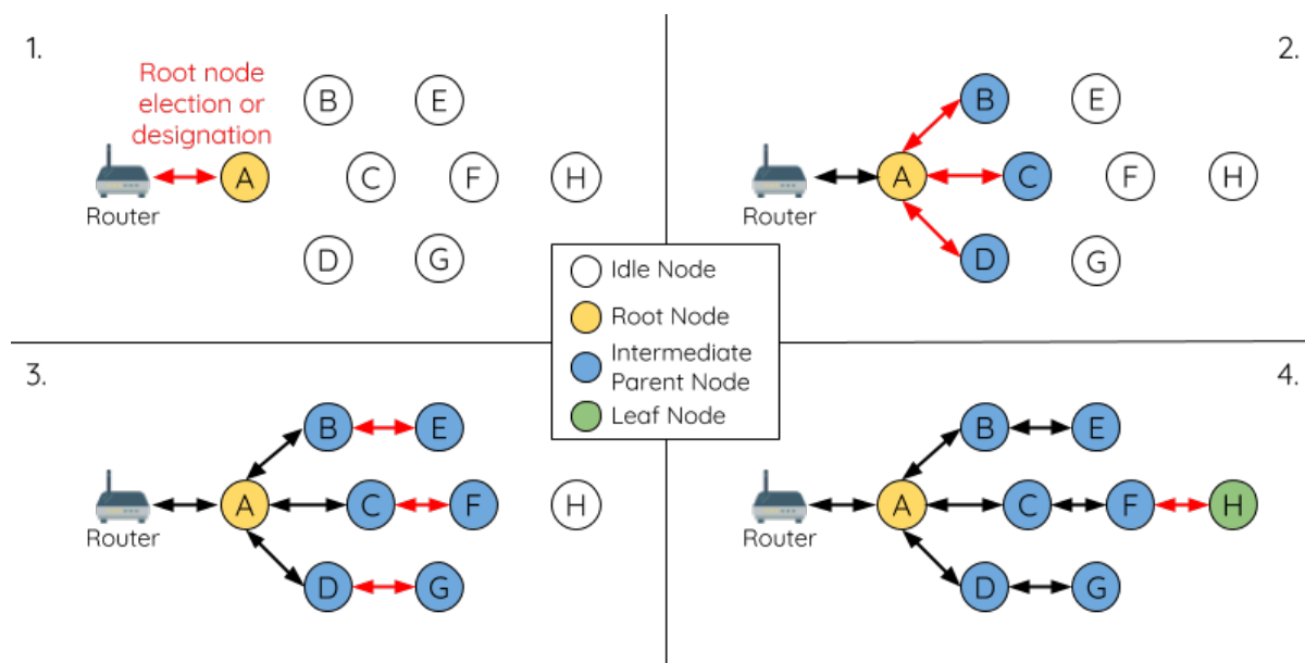
图 50: ESP-WIFI-MESH 网络构建过程
