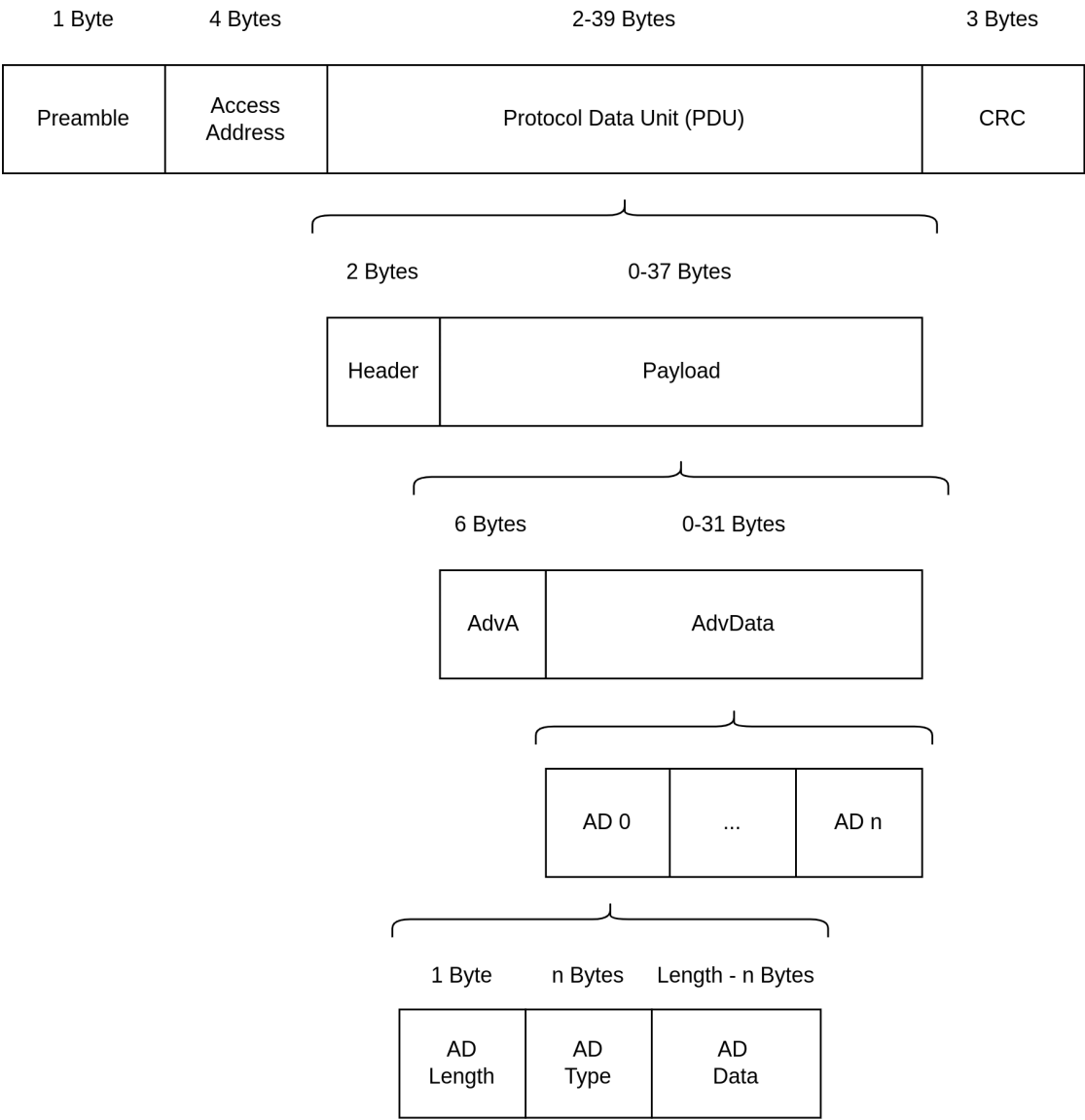
图 15: Bluetooth LE 4.2 广播数据包结构
