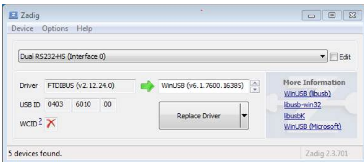
图 60: 在 Zadig 工具中配置 JTAG USB 驱动
