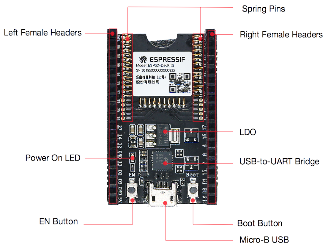
图 1: ESP32-DevKitS - 正面
