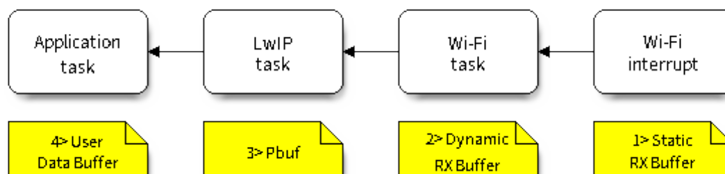
图 87: 接收数据缓冲区分配
