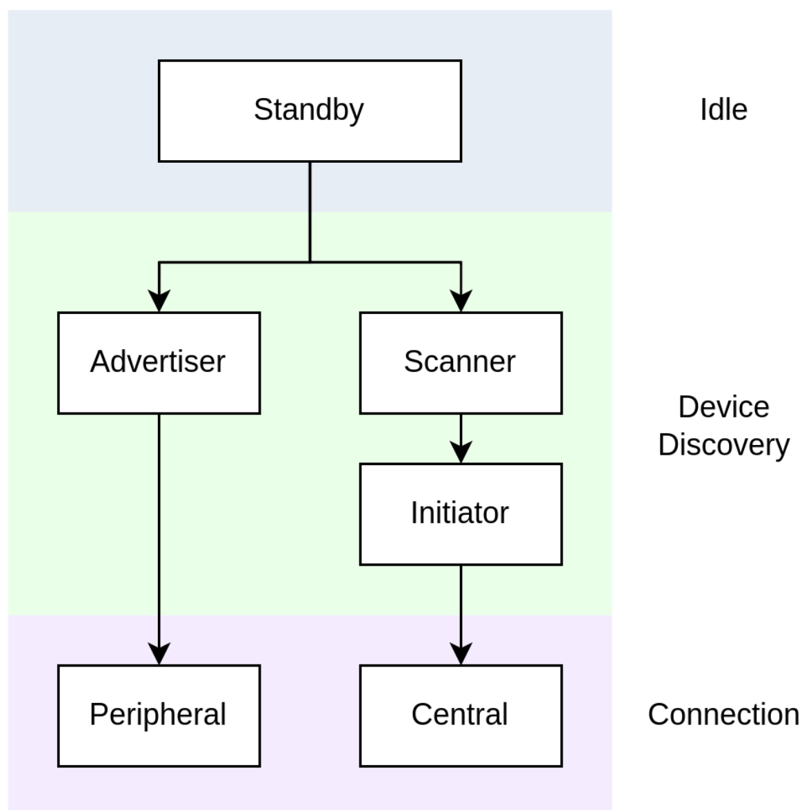
图 5: GAP 角色转换关系
