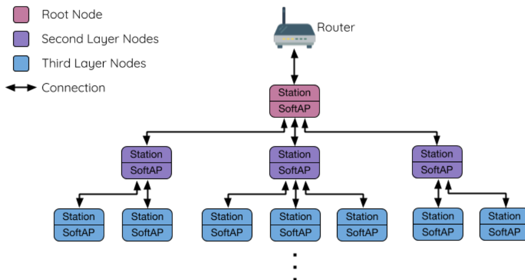
图 45: ESP-WIFI-MESH 树型拓扑
