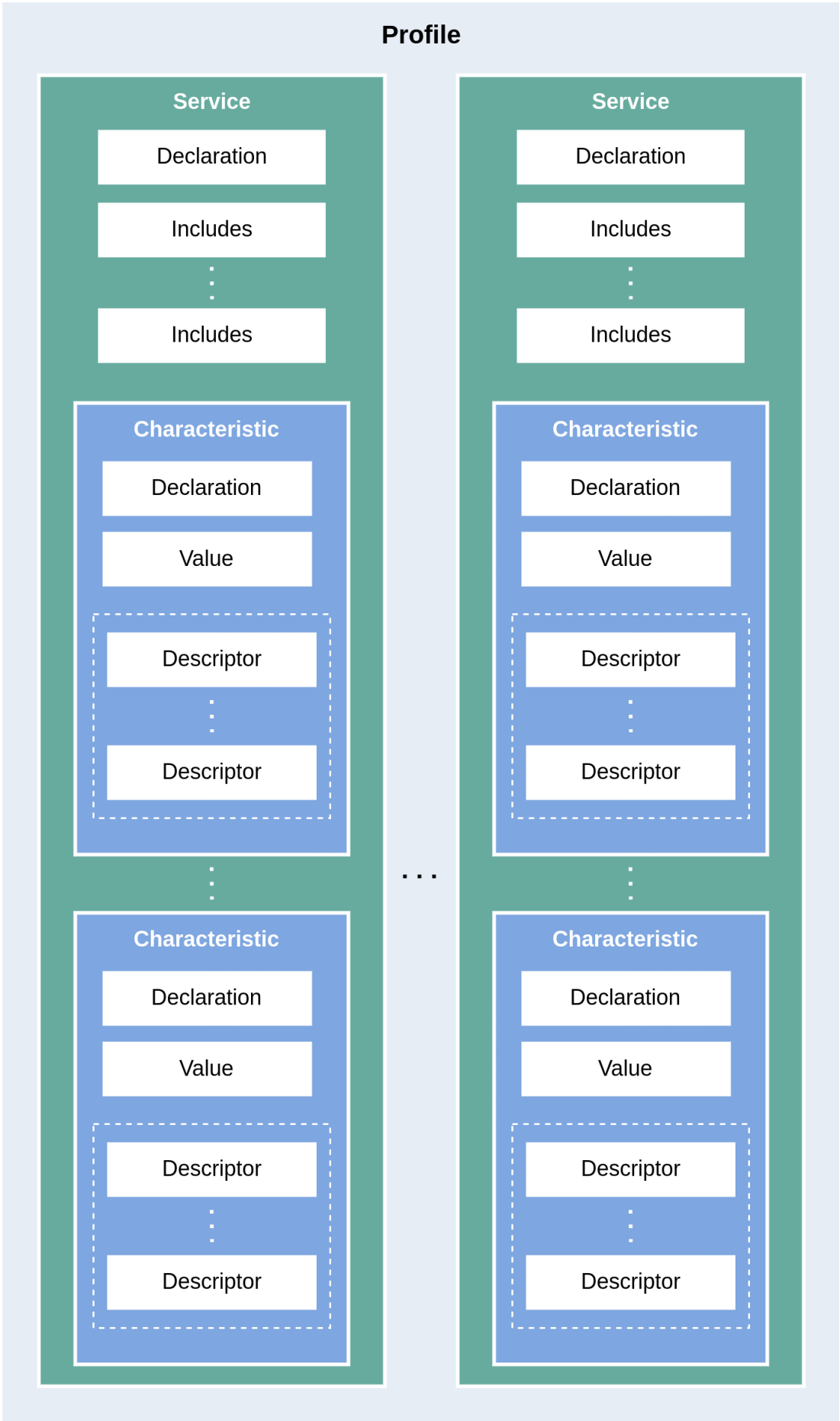
图 6: GATT 中的层次关系
