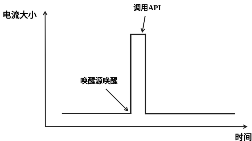
图 102: Deep-sleep 模式理想电流图
