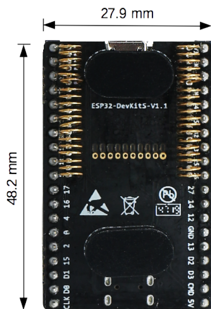
图 4: ESP32-DevKitS-R 尺寸 - 背面
