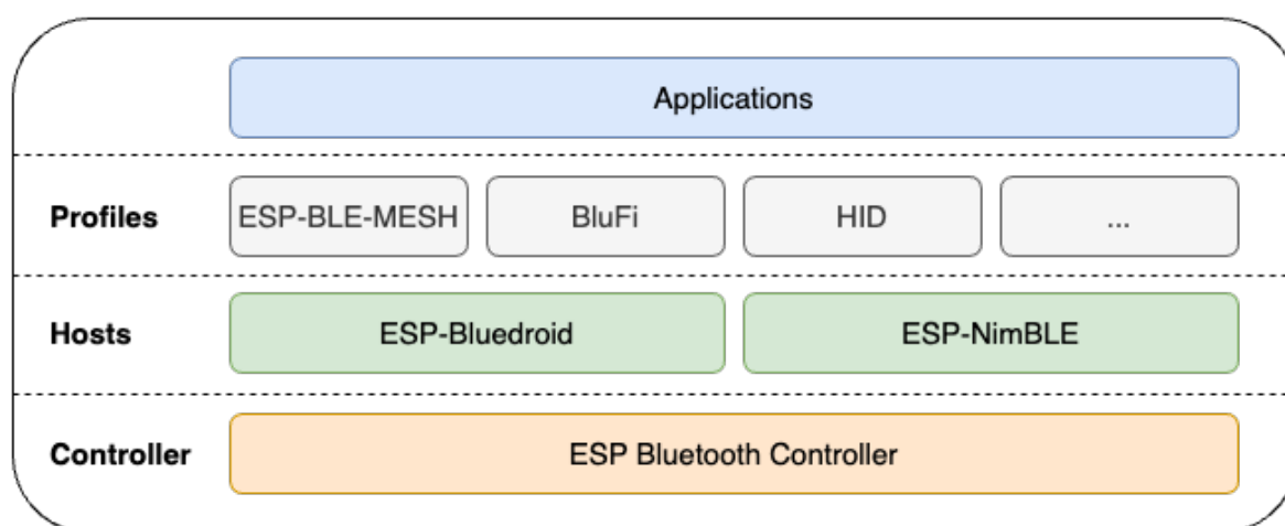
图 3: ESP32 蓝牙协议栈架构
