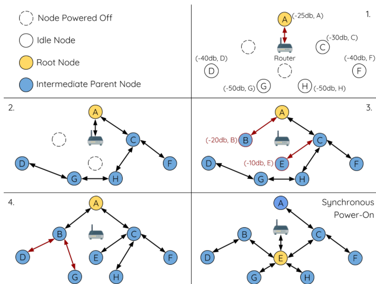
图 53: 网络构建（异步电源）示例
