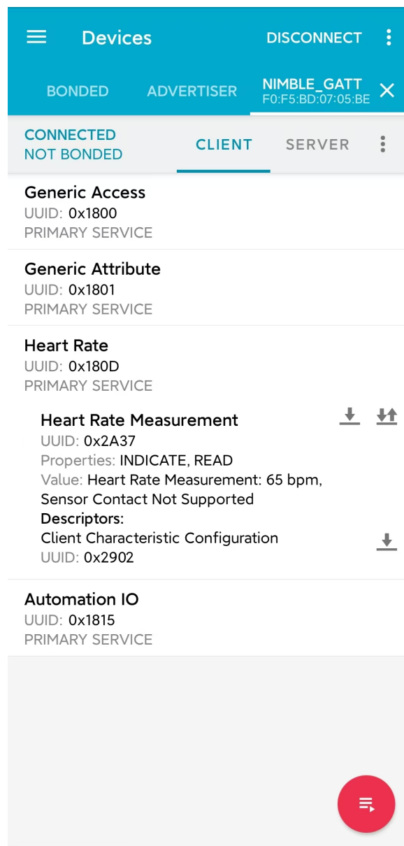
图 13: 对心率特征数据进行读访问
