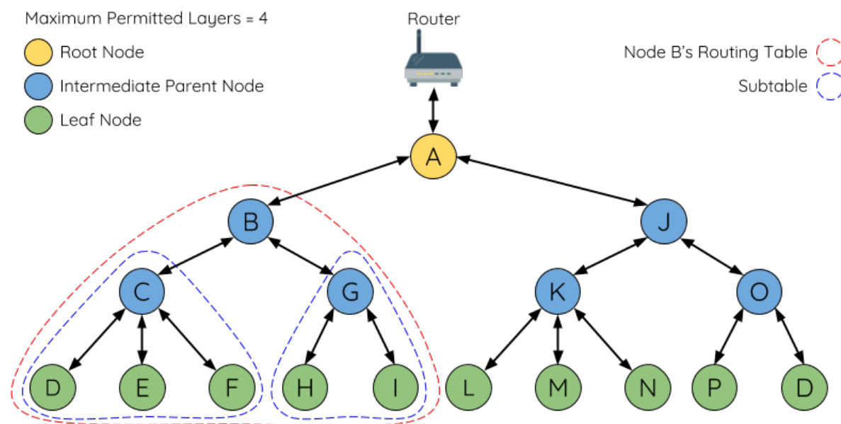
图 49: ESP-WIFI-MESH 路由表示例
