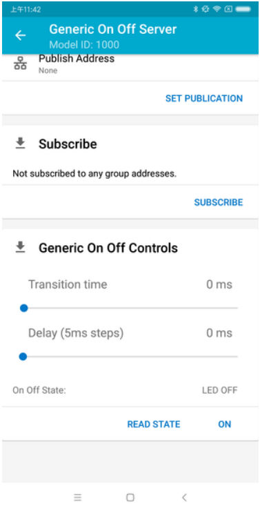
图 32: nRF Mesh - 通用开关控制
