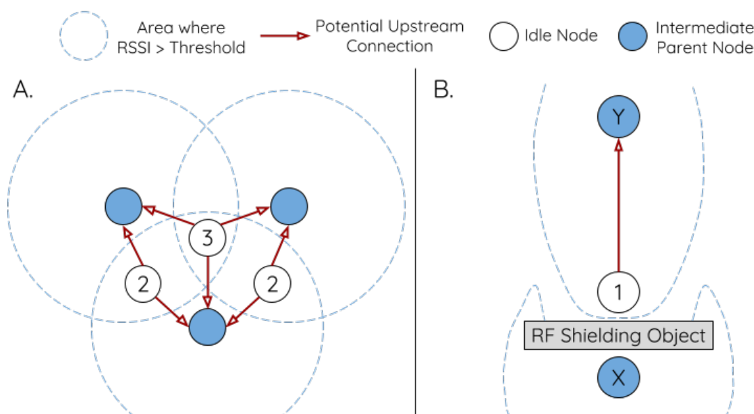
图 47: RSSI 阈值的影响
