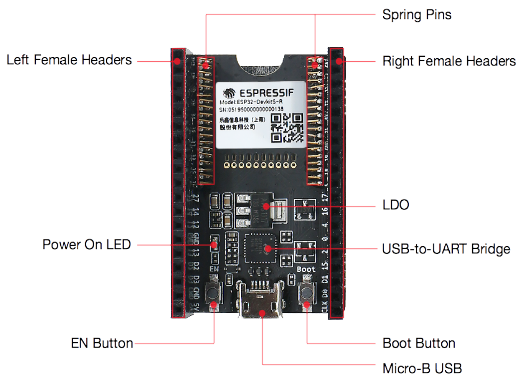
图 2: ESP32-DevKitS-R - 正面
