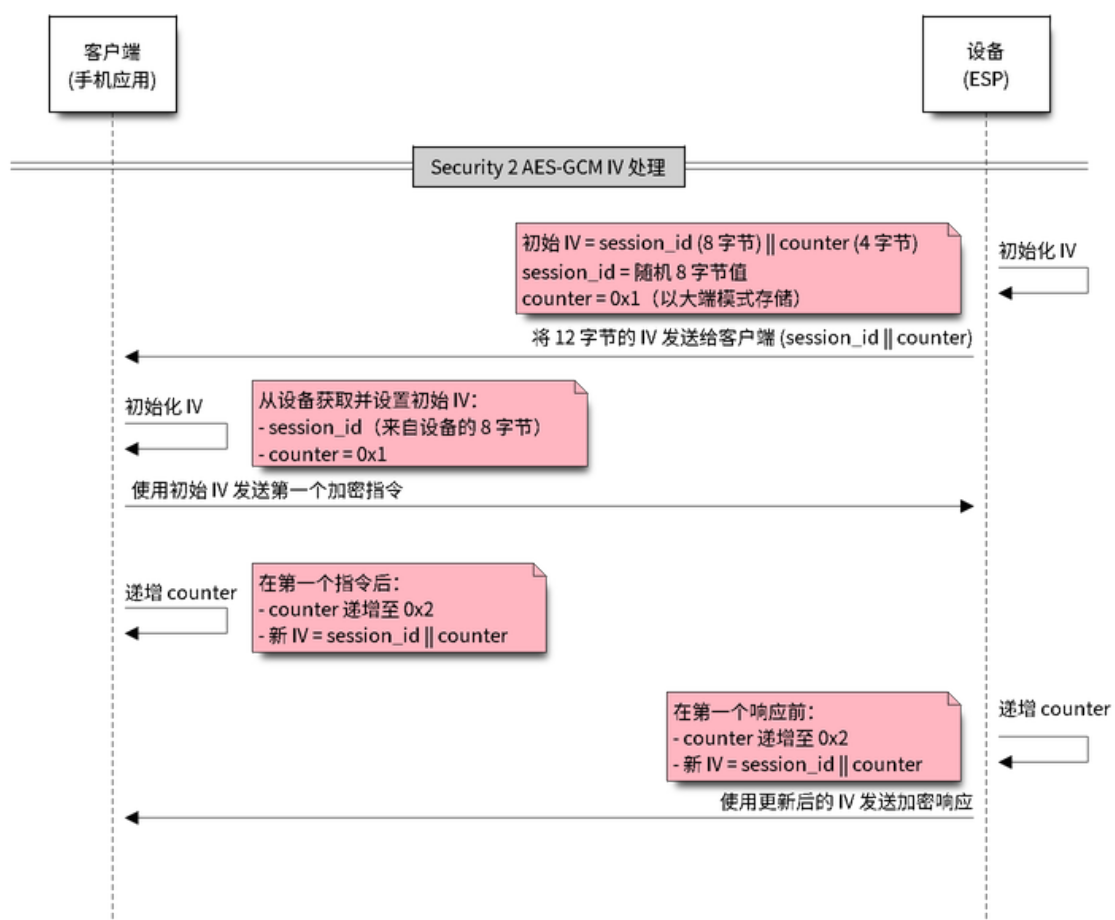
图 33: Security 2 AES-GCM IV 处理
