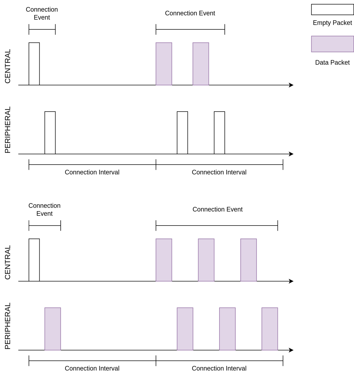
图 21: 连接间隔与连接事件
