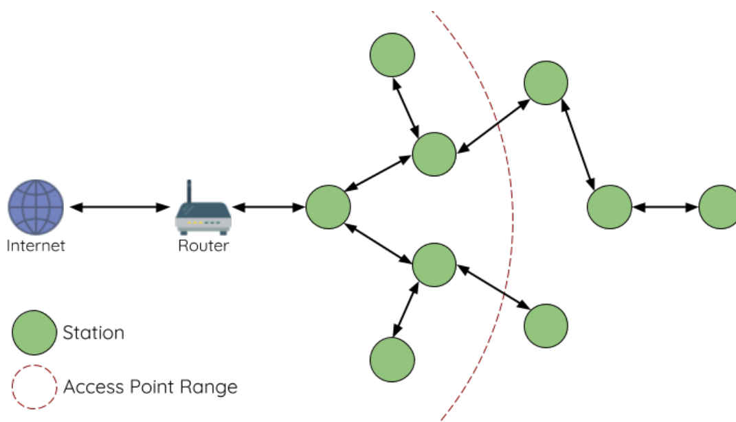
图 44: ESP-WIFI-MESH 网络架构示意图
