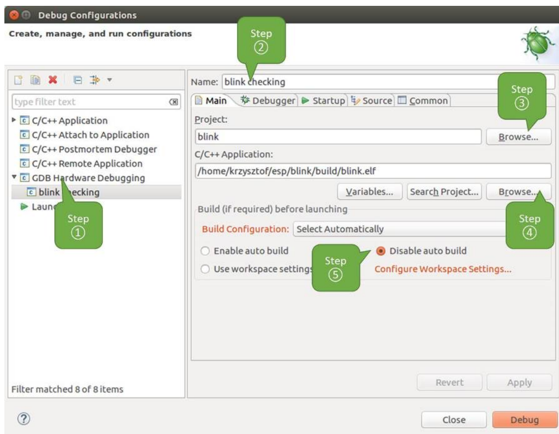
图 61: GDB 硬件调试的配置 - Main 选项卡
