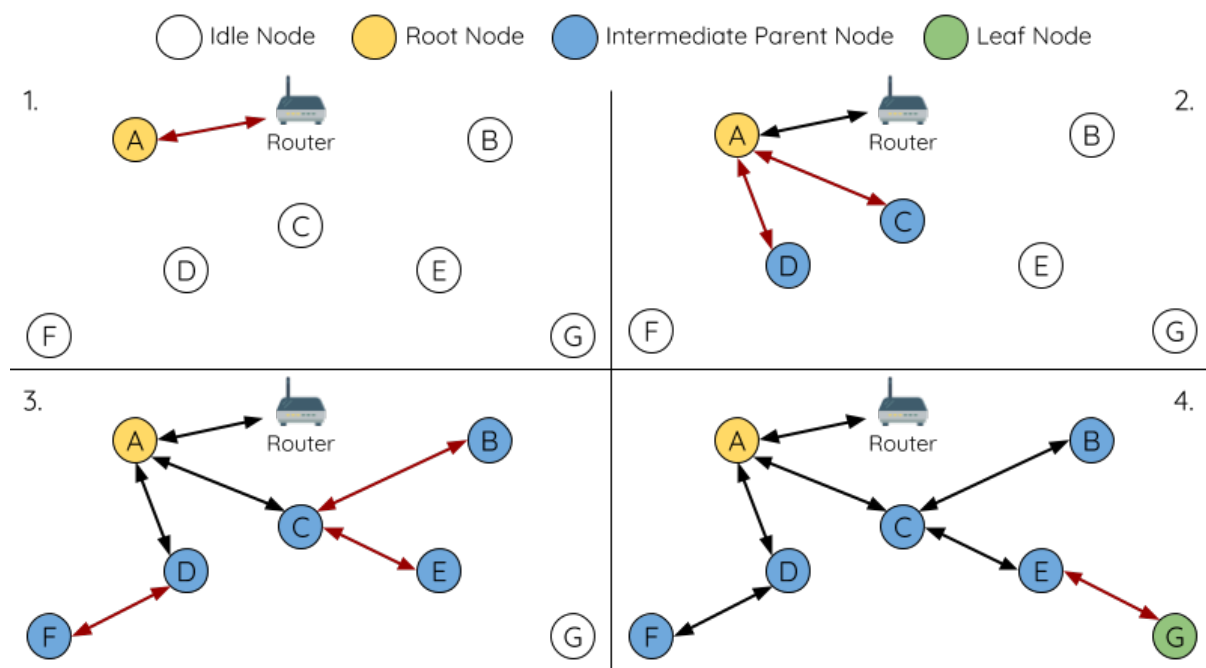
图 52: 根节点指定示例 (根节点 = A, 最大层级 = 4)
