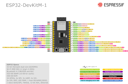
图 8: ESP32-DevKitM-1（点击放大）
