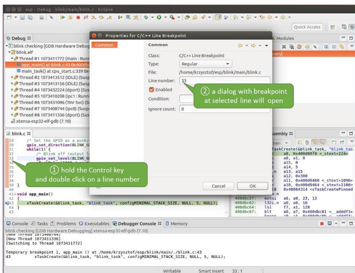
图 68: 设置断点
