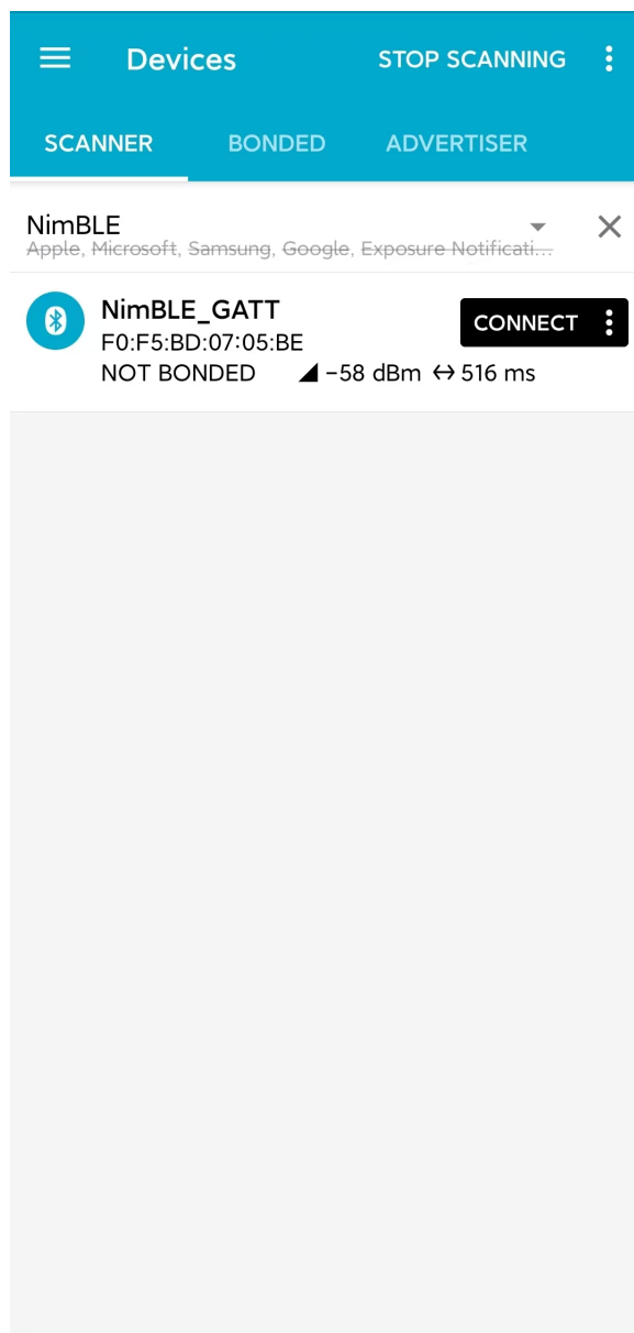
图 7: 扫描设备
