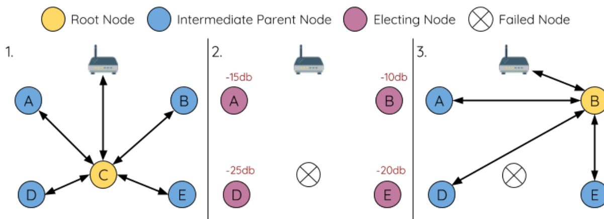
图 54: 根节点故障的自修复示意
