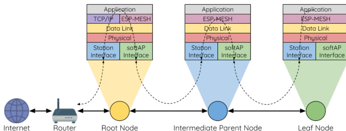
图 57: ESP-WIFI-MESH 双向数据流
