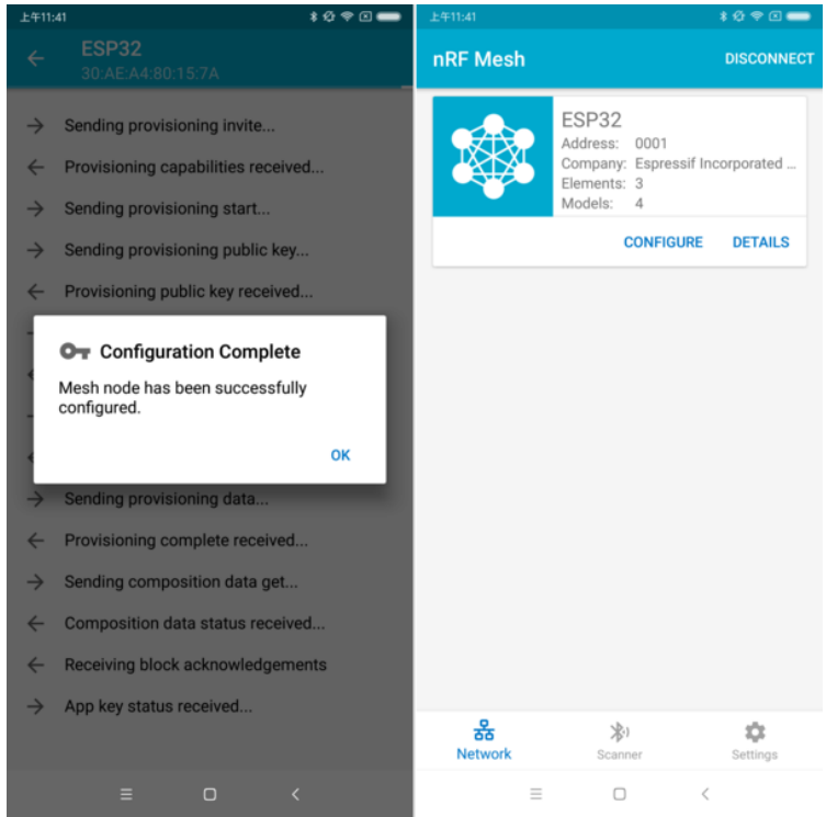
图 27: nRF Mesh - 配置完成
