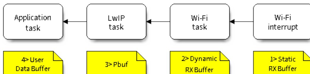
图 38: 接收数据缓冲区分配
