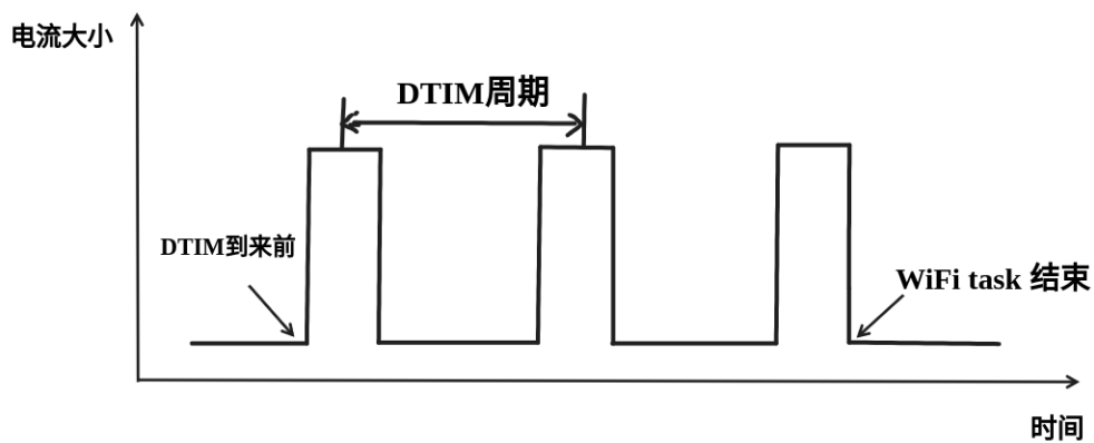
图 58: Min Modem-sleep 理想电流图
