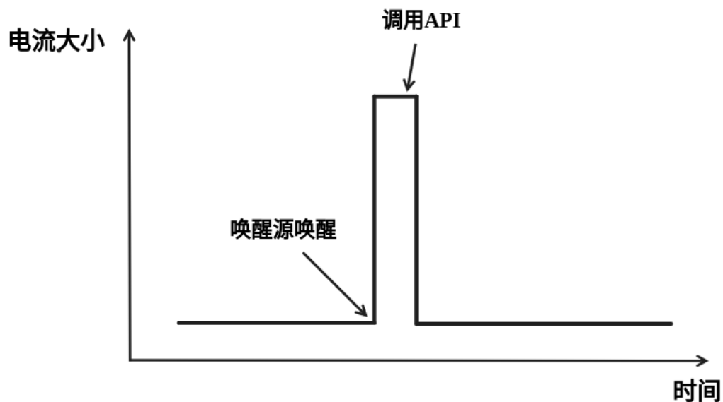
图 53: Deep-sleep 模式理想电流图
