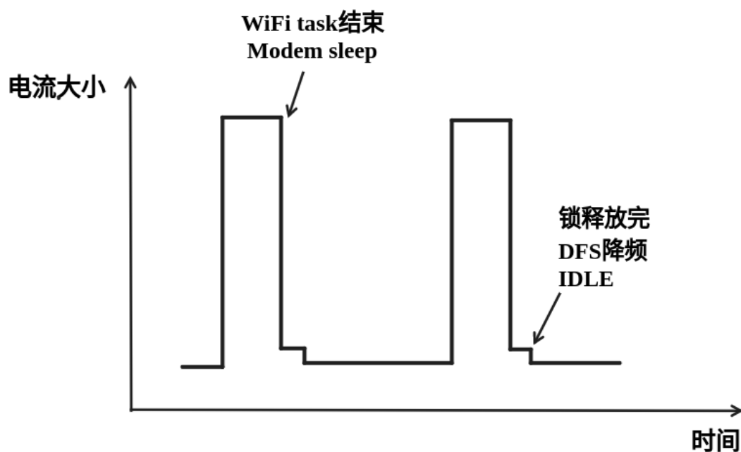
图 60: DFS+Modem sleep 模式理想电流图
