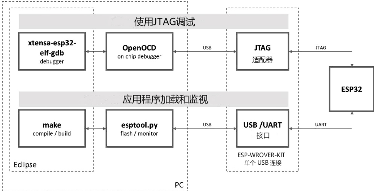
图 11: JTAG 调试 - 概述图
