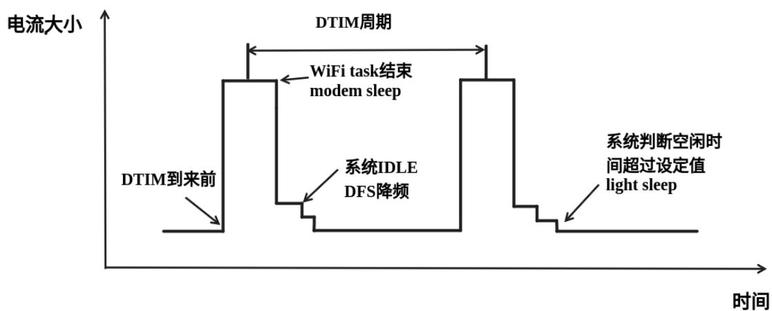
图 62: modem+auto light-sleep 模式理想电流图
