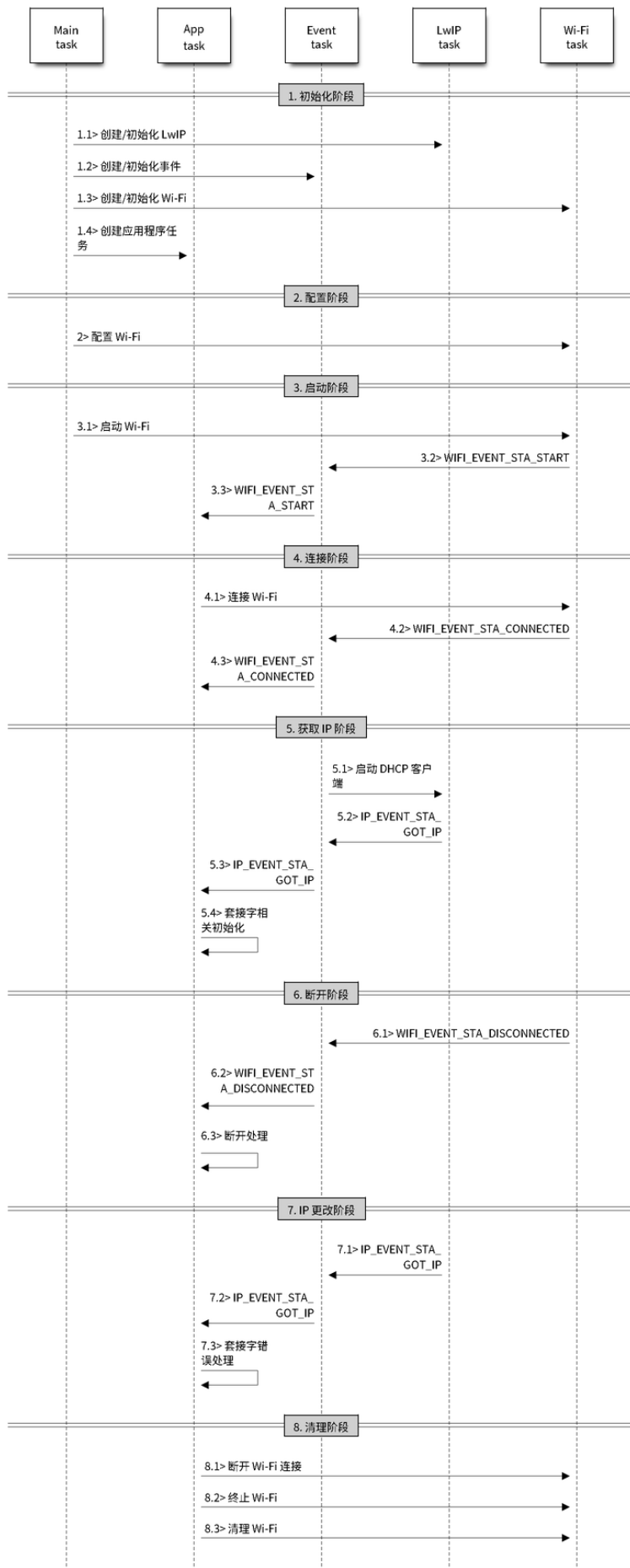
图 30: station 模式下 Wi-Fi 事件场景示例
