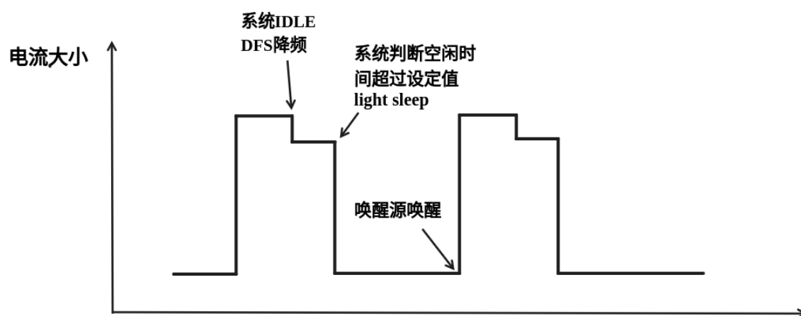
图 51: Auto Light-sleep 模式模式理想电流图
