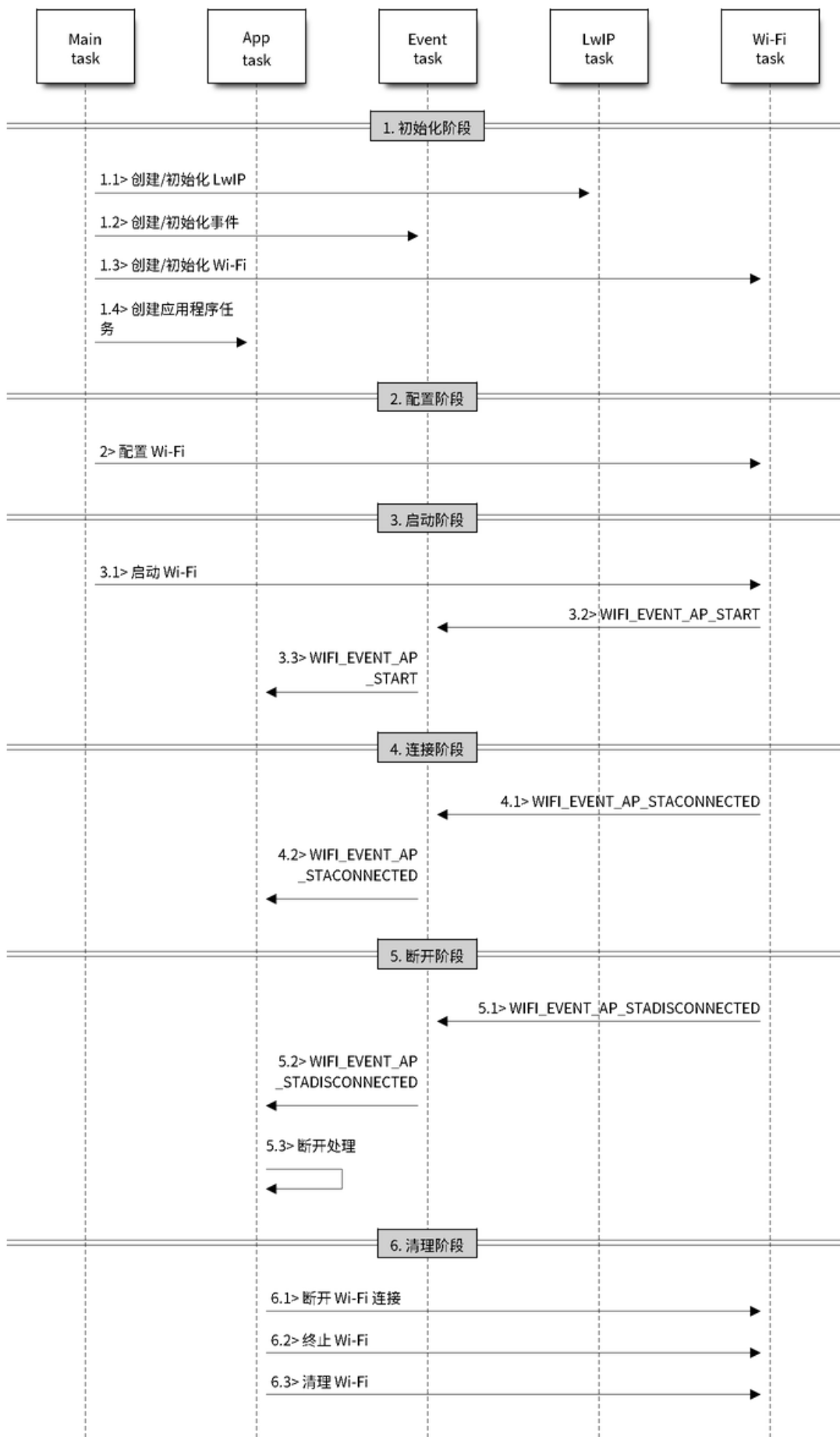
图 31: AP 模式下 Wi-Fi 事件场景示例
