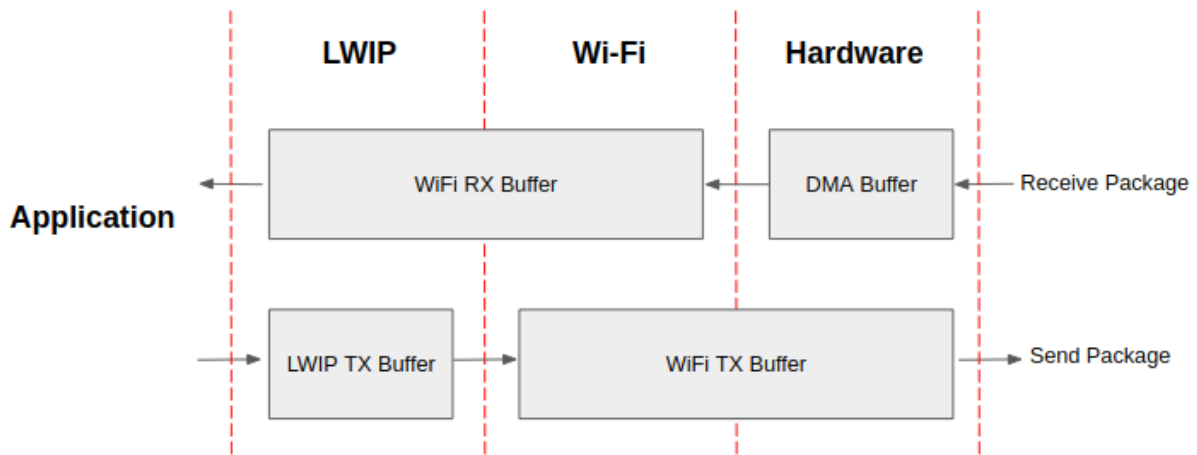
图 36: ESP32-C2 数据路径
