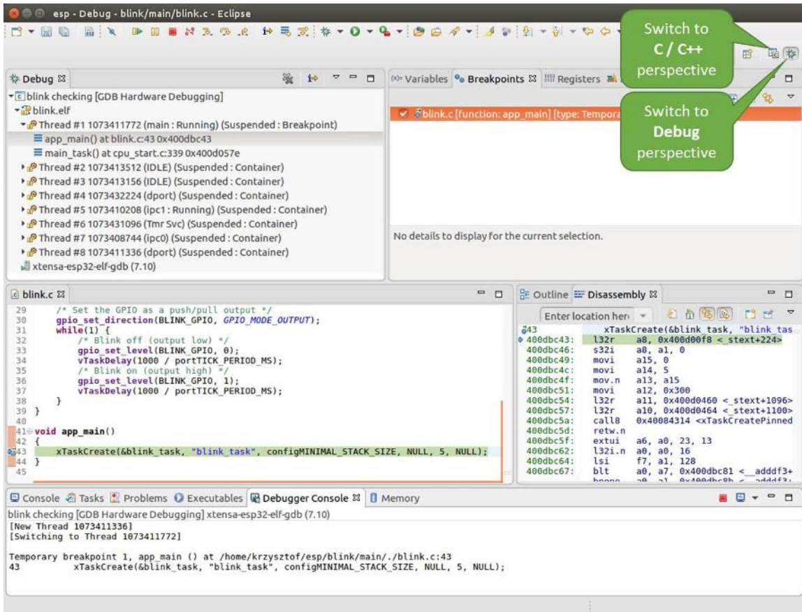
图 15: Eclipse 中的调试视图
