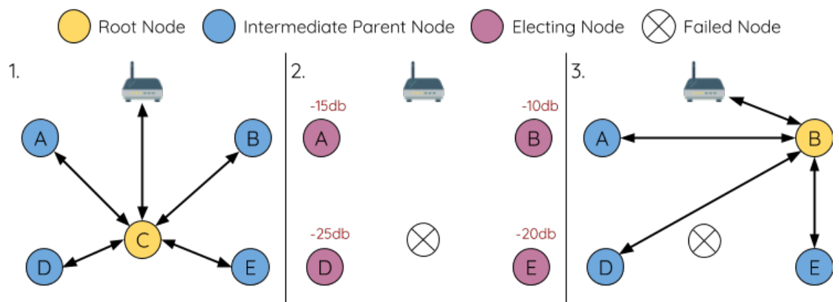
图 33: 根节点故障的自修复示意
