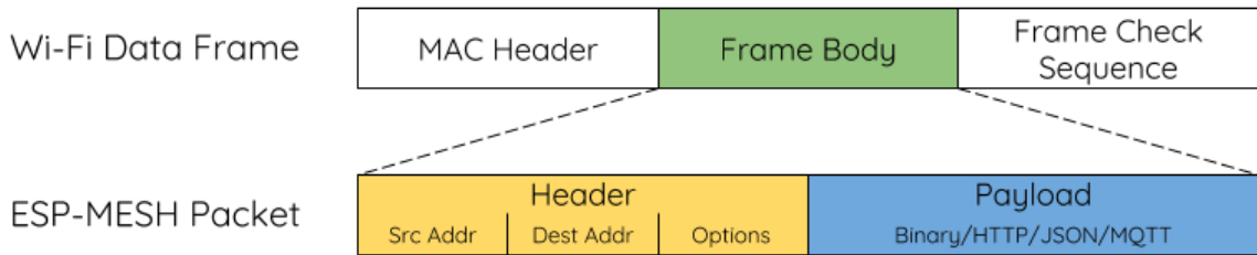
图 55: ESP-WIFI-MESH 数据包
