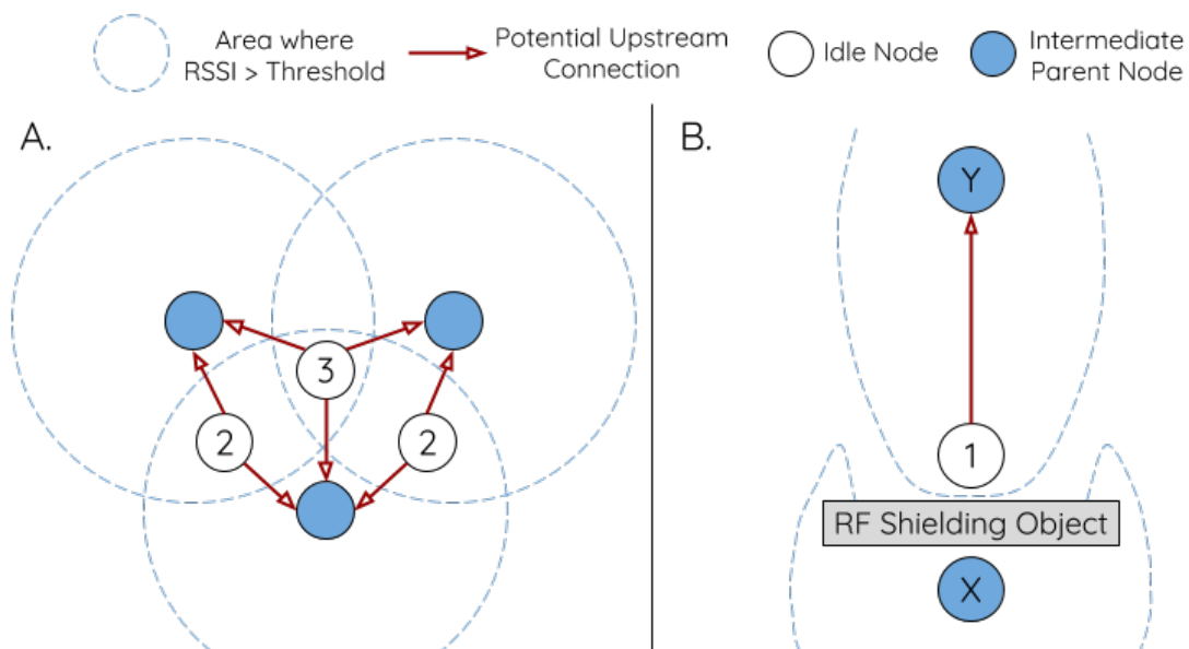
图 46: RSSI 閾值的影响
