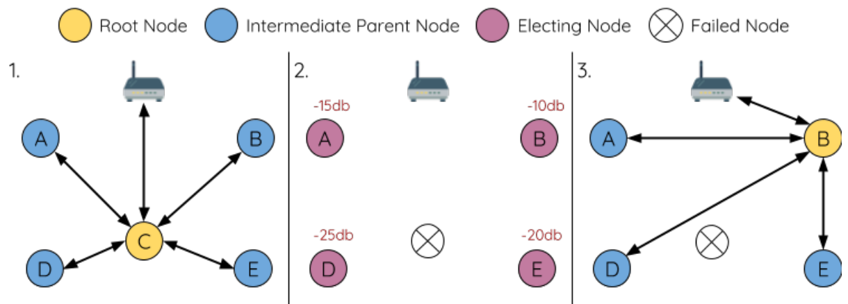
图 53: 根节点故障的自修复示意
