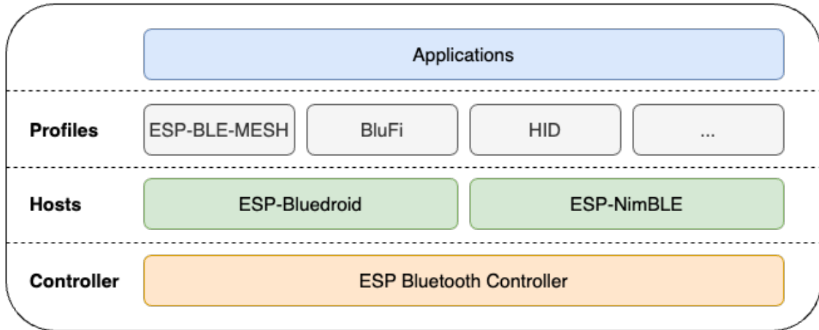
图 2: ESP32-C3 蓝牙协议栈架构
