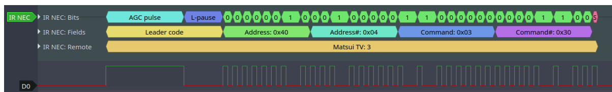
图 15: 红外 NEC 帧
