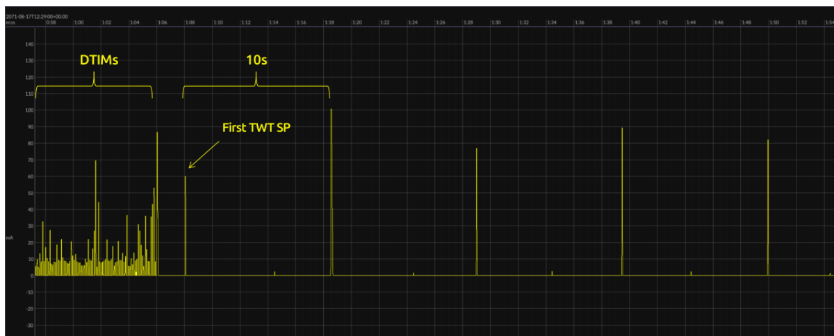
图 92: DTIM 与 iTWT 模式下的电流图
