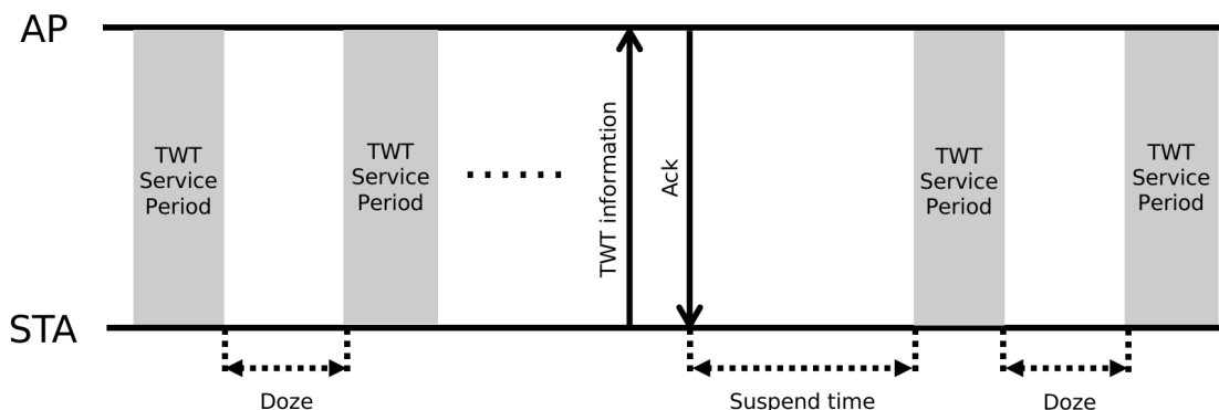
图 90: Individual TWT 协商暂停/恢复过程示例
