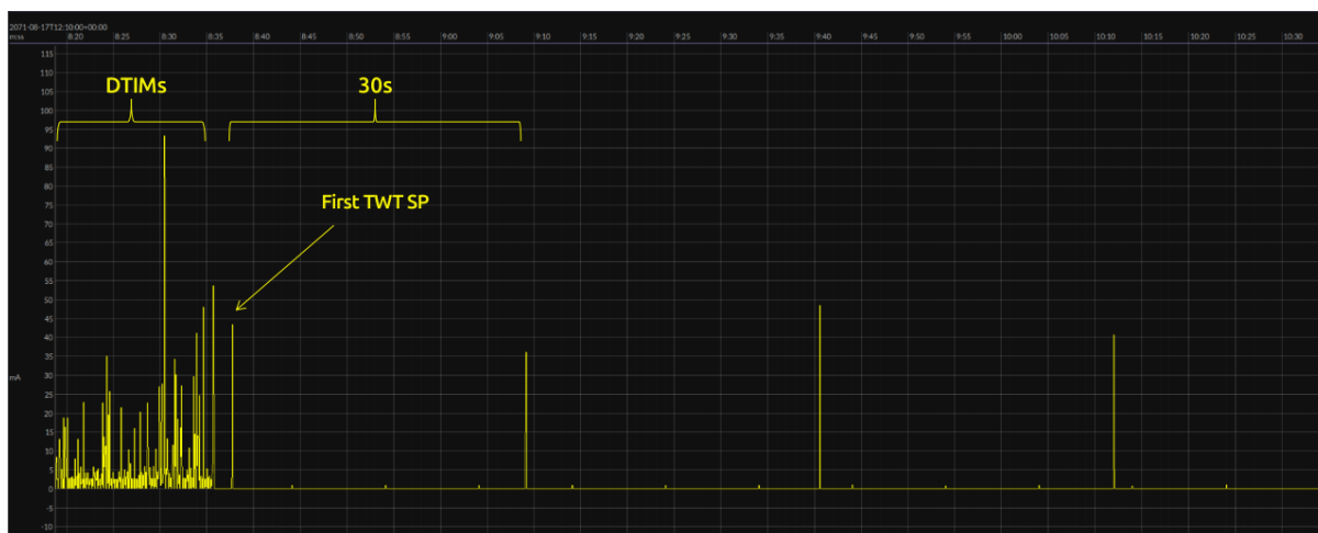
图 94: 更改参数后的 DTIM 与 iTWT 模式下的电流图
