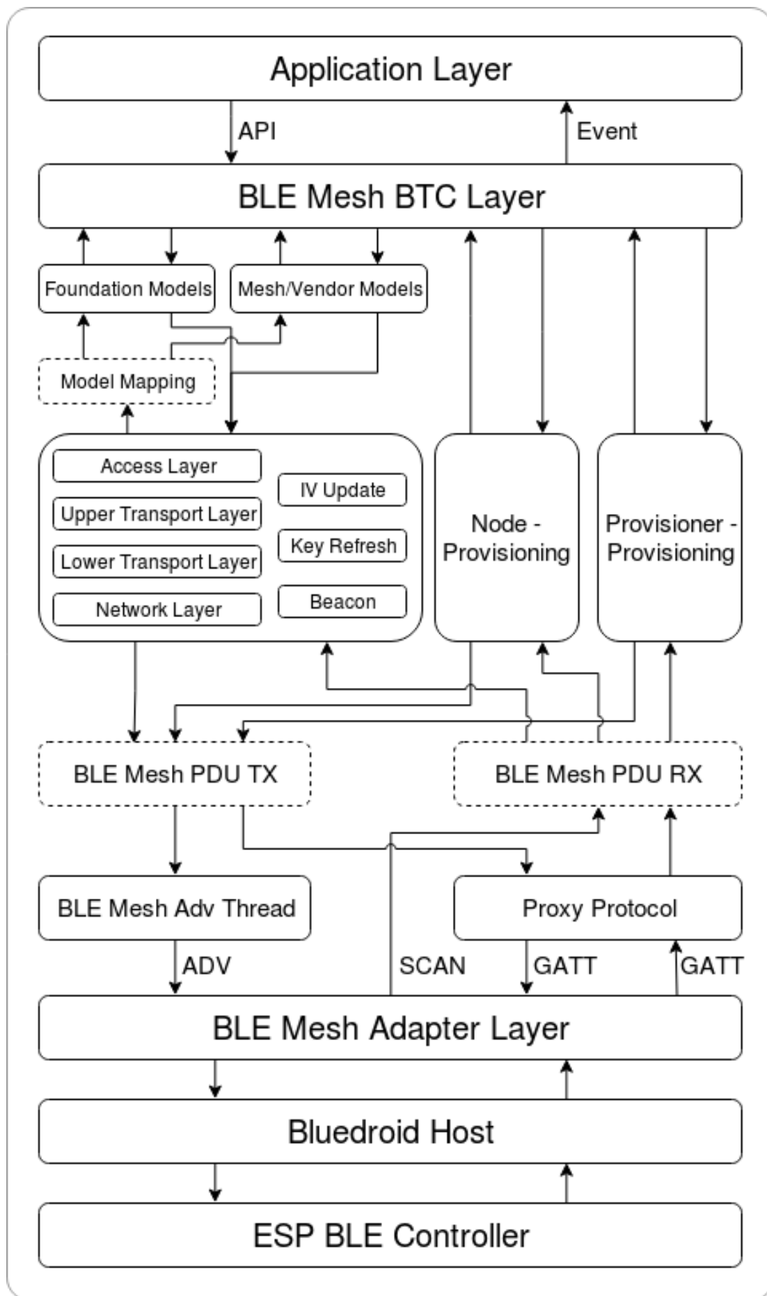
图 14: 图 2.1 ESP-BLE-MESH 架构实现图
