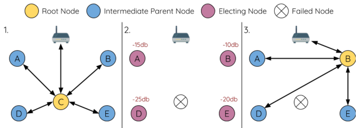
图 33: 根节点故障的自修复示意
