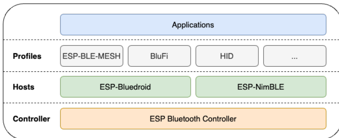
图 2: ESP32-C6 蓝牙协议栈架构
