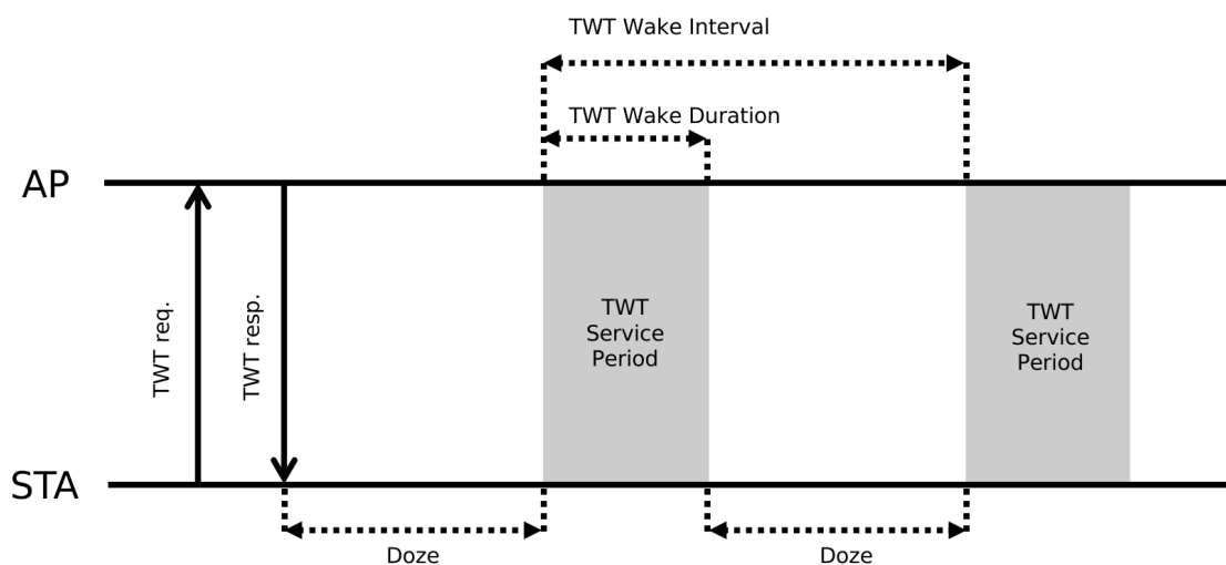
图 90: Individual TWT 协商建立过程示例
