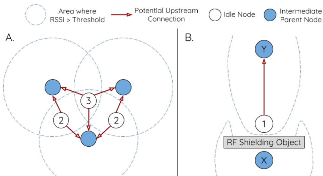
图 26: RSSI 阈值的影响
