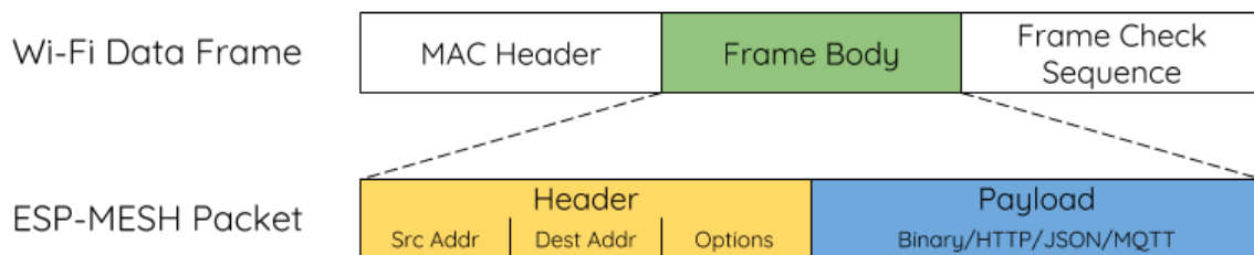
图 35: ESP-WIFI-MESH 数据包
