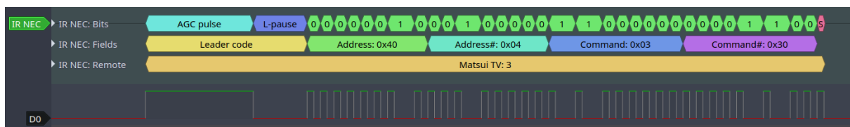
图 19: 红外 NEC 帧
