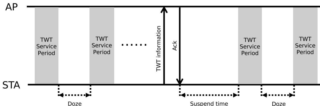
图 111: Individual TWT 协商暂停/恢复过程示例
