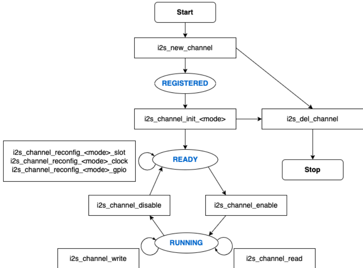
图 9: I2S 有限状态机
