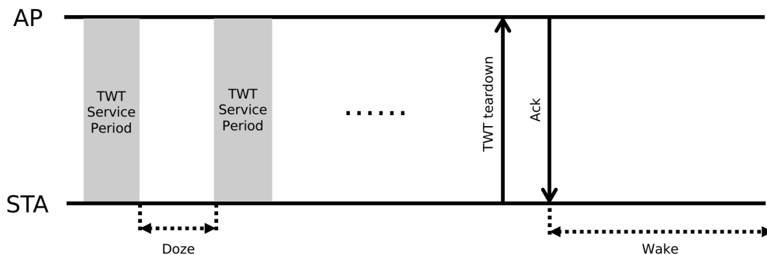
图 112: Individual TWT 协商终止过程示例
