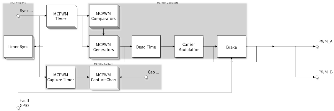
图 11: MCPWM Overview
