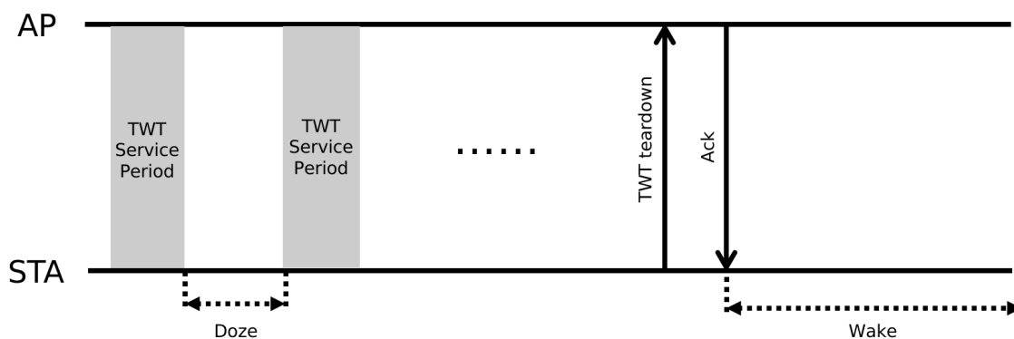
图 112: Individual TWT 协商终止过程示例
