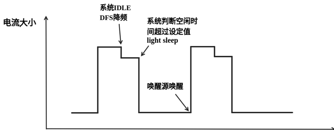
图 62: Auto Light-sleep 模式模式理想电流图
