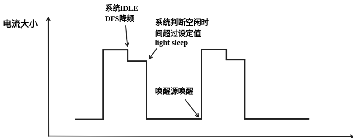
图 62: Auto Light-sleep 模式模式理想电流图
