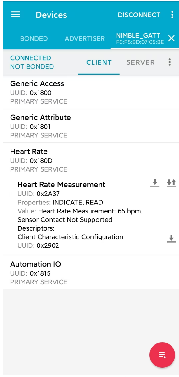
图 12: 对心率特征数据进行读访问
