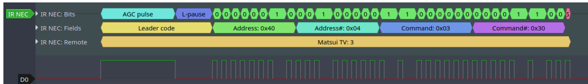
图 17: 红外 NEC 帧
