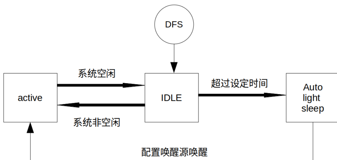
图 60: Auto Light-sleep 模式工作流程图
