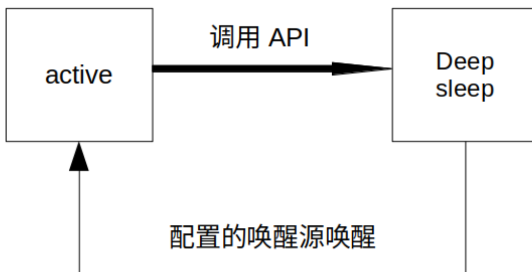
图 62: Deep-sleep 模式工作流程图
