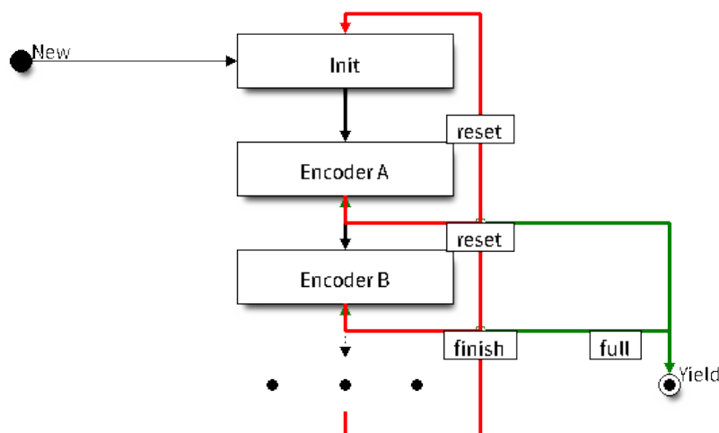
图 16: RMT 编码器链
