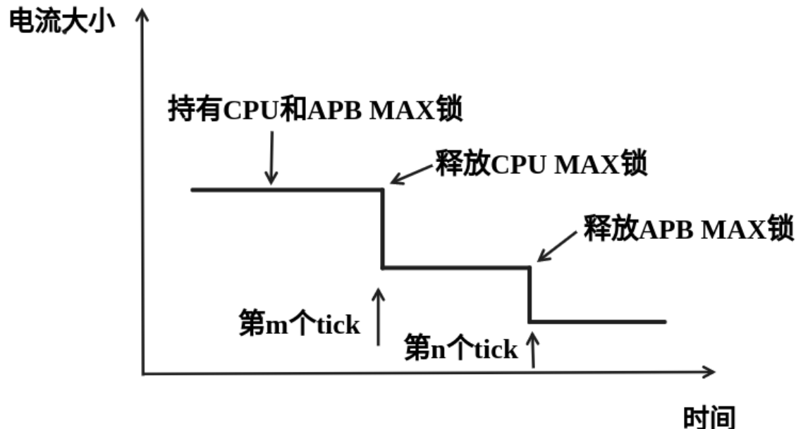
图 59: 理想 DFS 机制调频电流图
