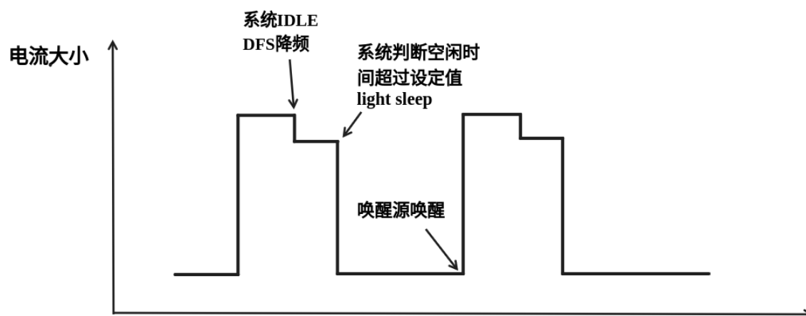
图 61: Auto Light-sleep 模式理想电流图
