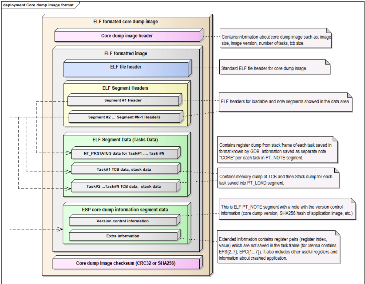
图 37: 核心转储 ELF 镜像文件格式
