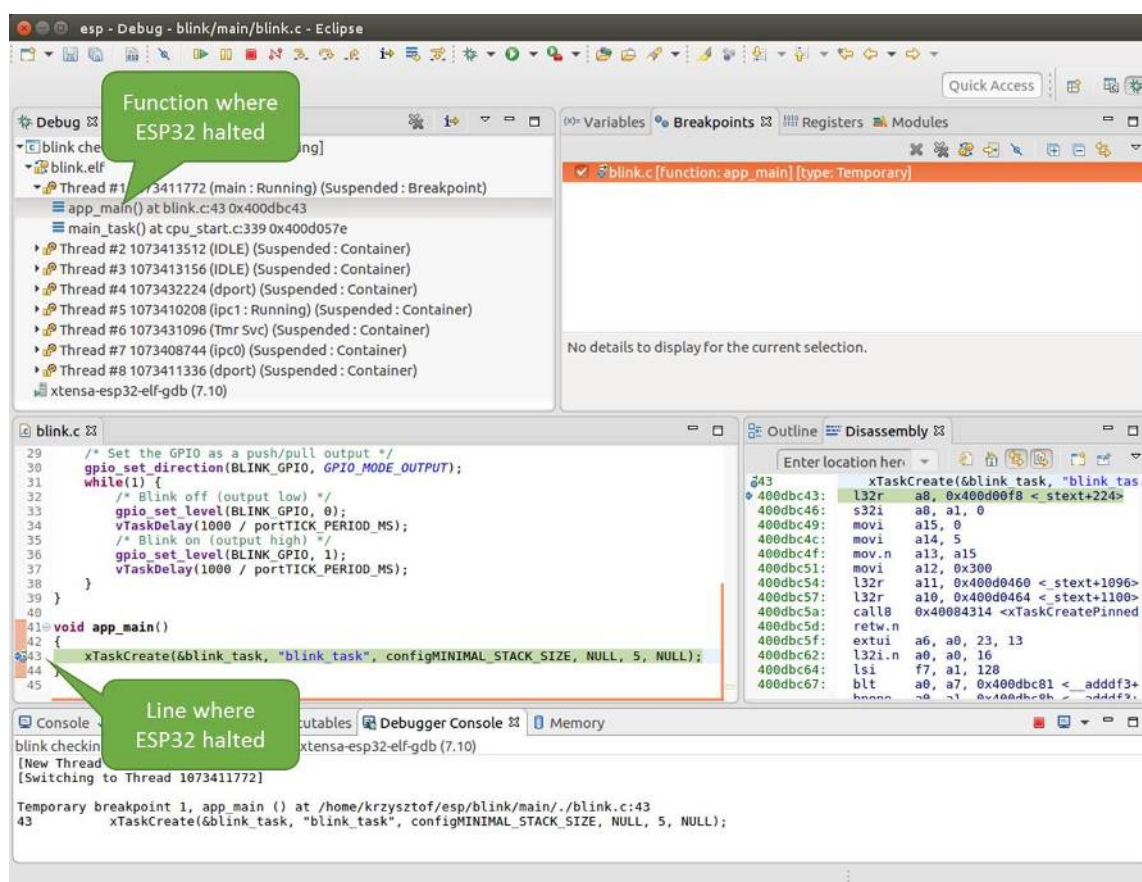
图 47: 调试时目标停止
