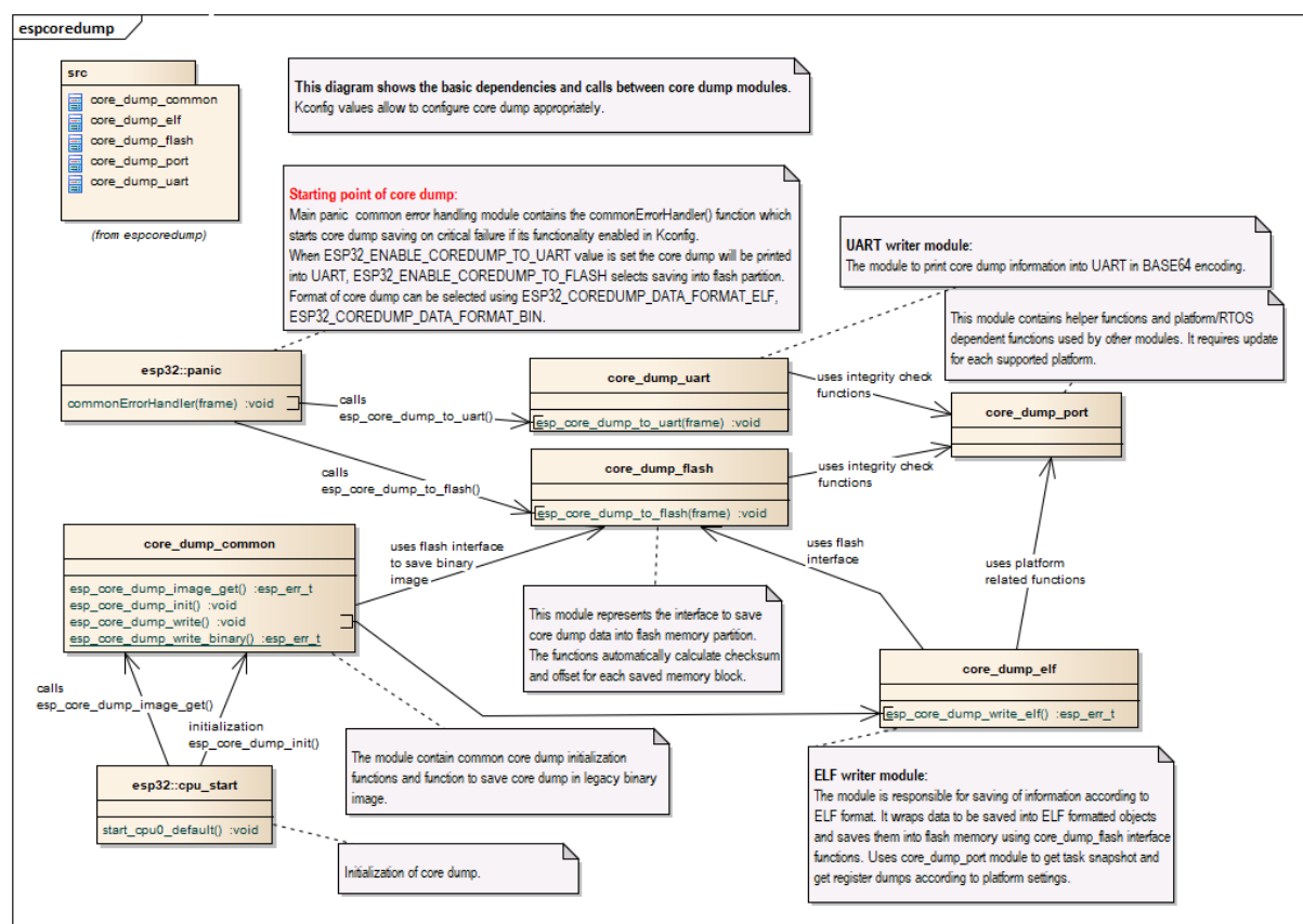
图 39: 核心转储实现
