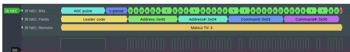
图 17: 红外 NEC 帧
