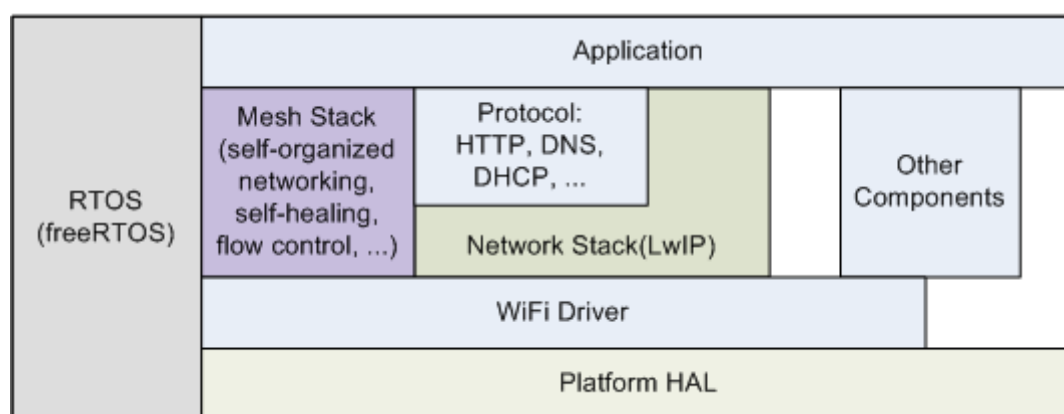
图 1: ESP-WIFI-MESH 软件栈
