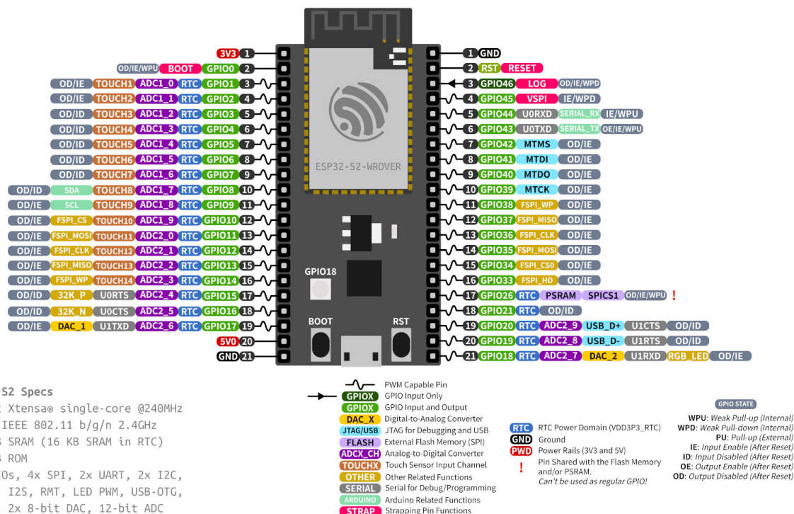
图 4: ESP32-S2-Saola-1 管脚布局 (点击放大)
