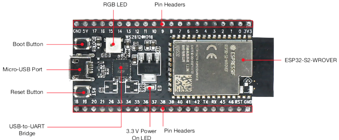
图 2: ESP32-S2-Saola-1 - 正面
