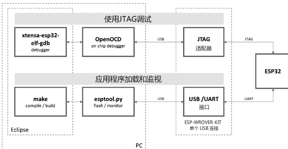
图 37: JTAG 调试 - 概述图
