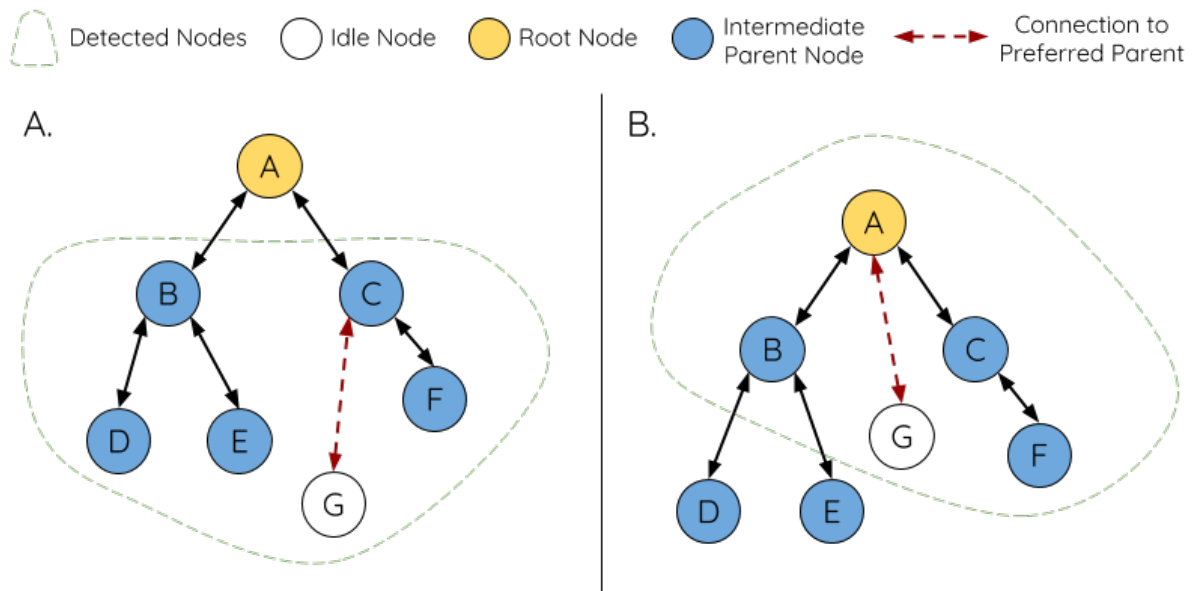
图 27: 首选父节点选择
