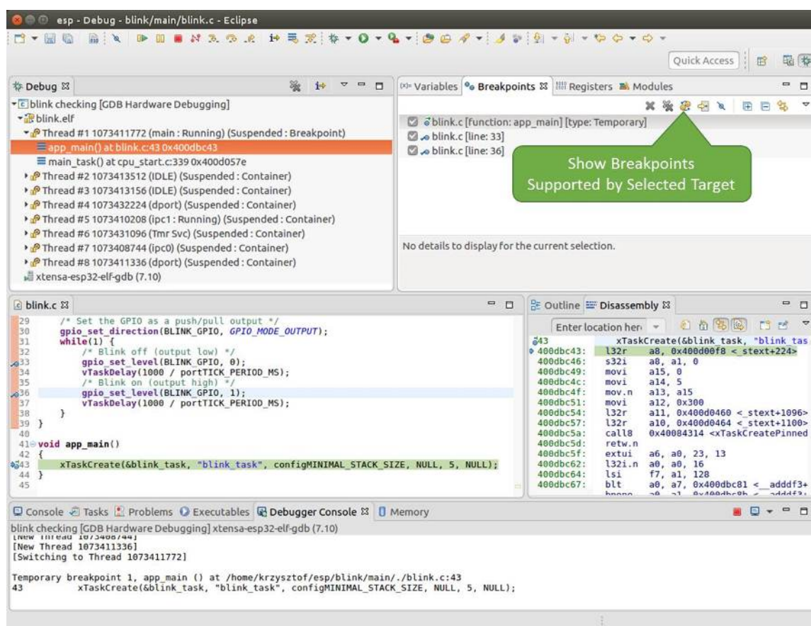
图 67: 设置了三个断点 / 最多允许两个断点
