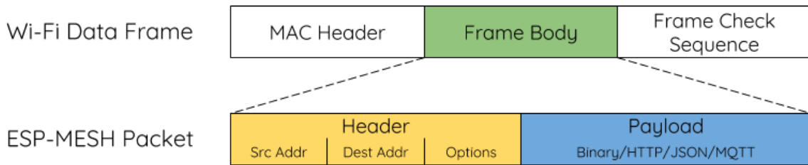
图 55: ESP-WIFI-MESH 数据包
