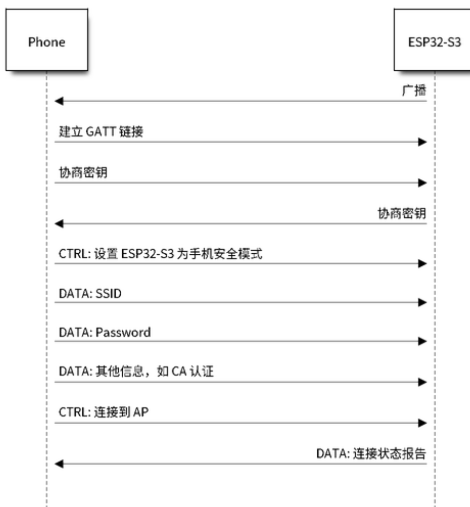
图 35: BluFi Flow Chart
