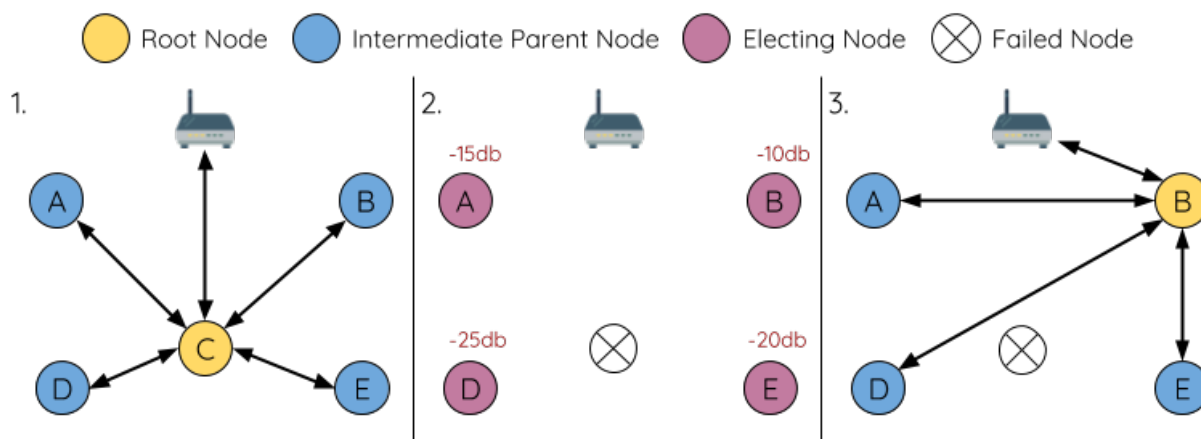
图 53: 根节点故障的自修复示意
