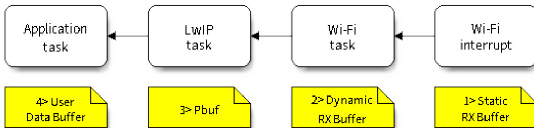
图 88: 接收数据缓冲区分配
