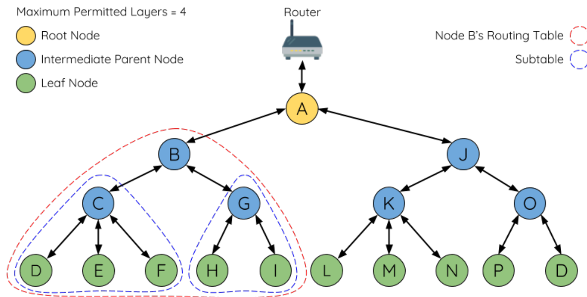
图 31: ESP-WIFI-MESH 路由表示例
