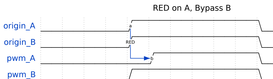
PWMA 上升沿延迟, 绕过PWMB 死区
