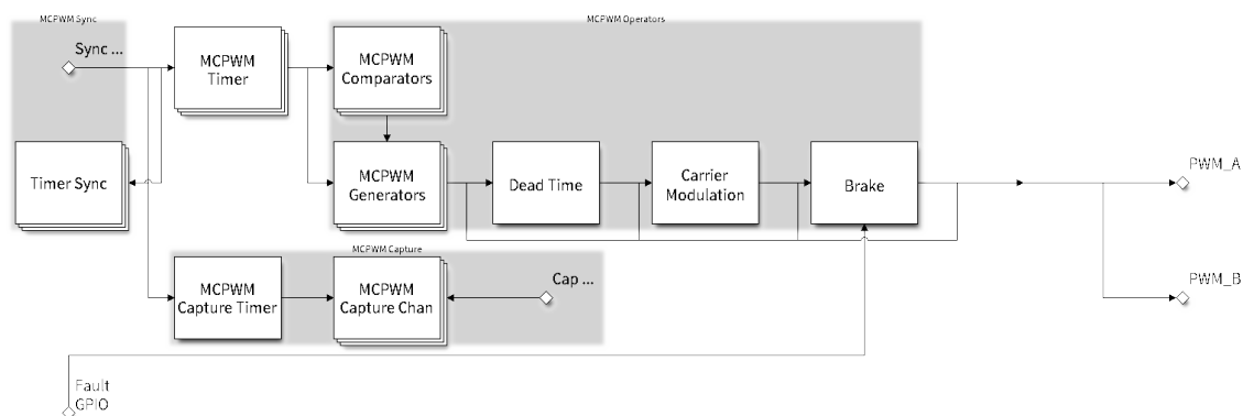
图 16: MCPWM 概述
