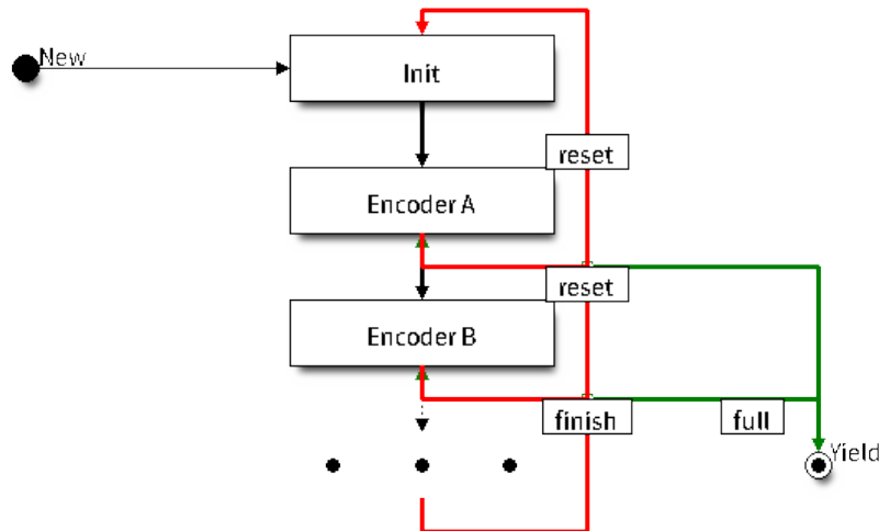
图 25: RMT 编码器链
