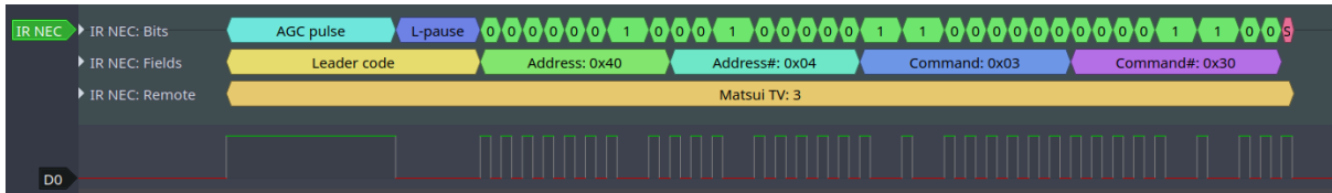
图 26: 红外 NEC 帧
