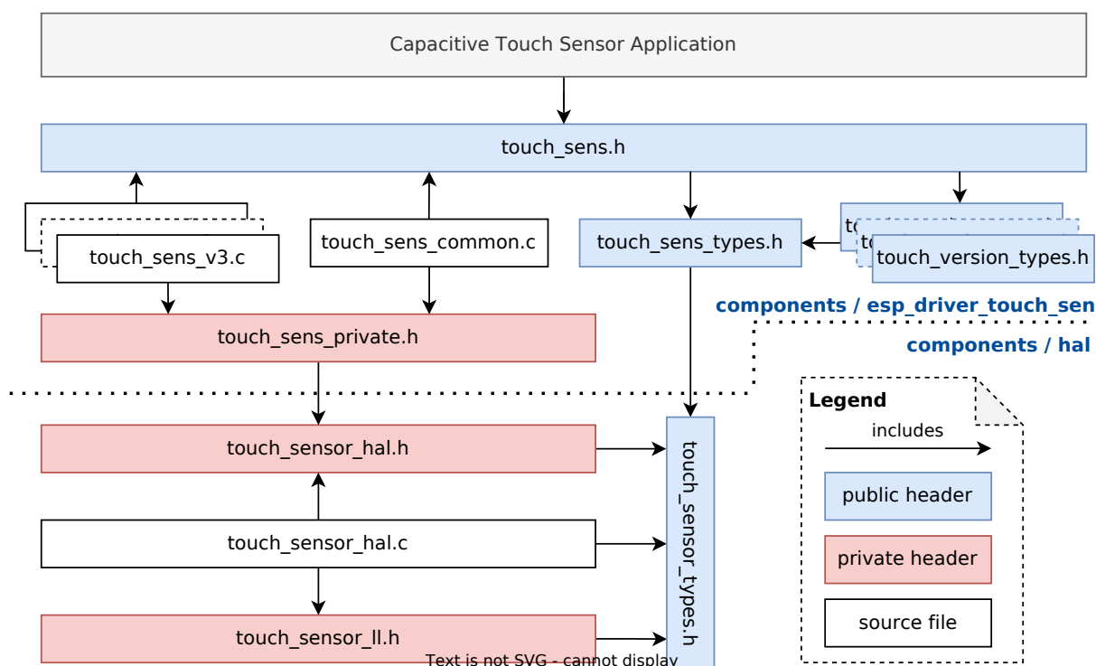
图 37: 触摸传感器驱动文件结构图
