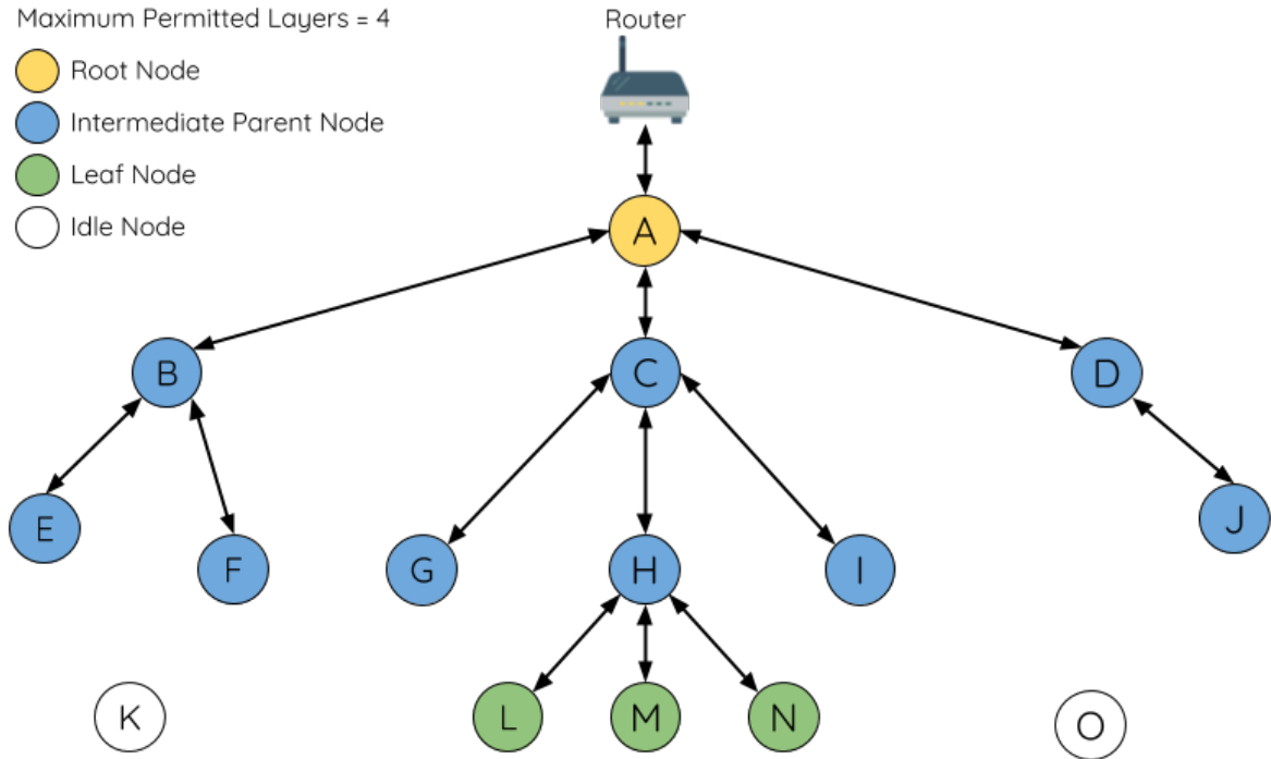
图 29: ESP-WIFI-MESH 节点类型
