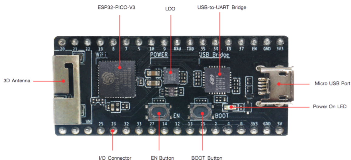
图 13: ESP32-PICO-KIT-1 开发板布局 - 正面 (点击放大)
