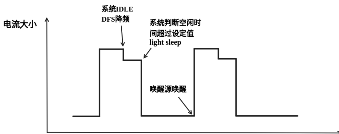
图 83: Auto Light-sleep 模式模式理想电流图
