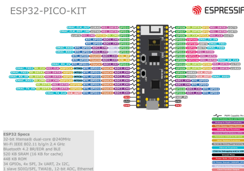
图 3: ESP32-PICO-KIT 管脚布局 (点击放大)
