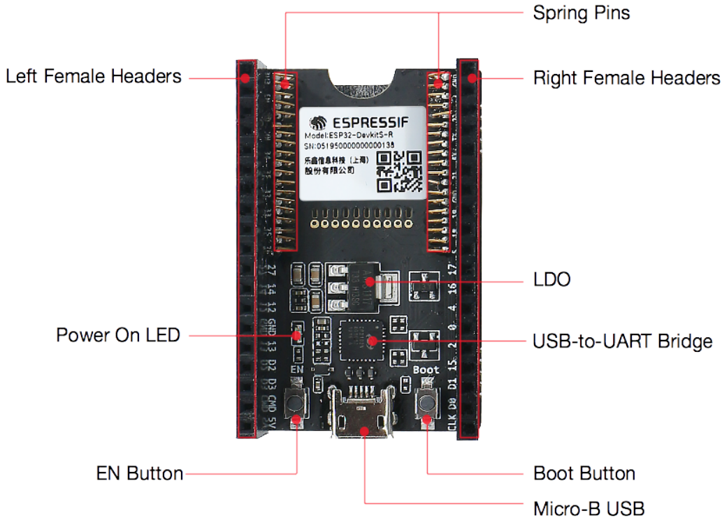
图 8: ESP32-DevKitS-R - 正面
