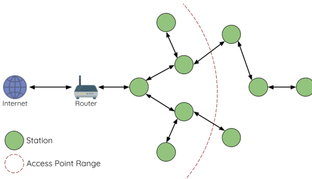
图 27: ESP-WIFI-MESH 网络架构示意图
