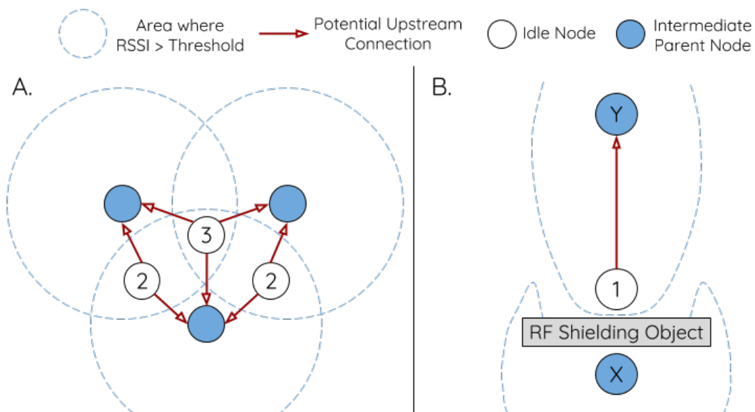
图 30: RSSI 閾值的影响
