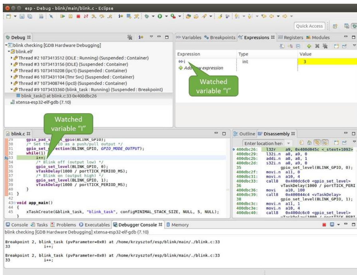
图 58: 观察程序变量 “i”
