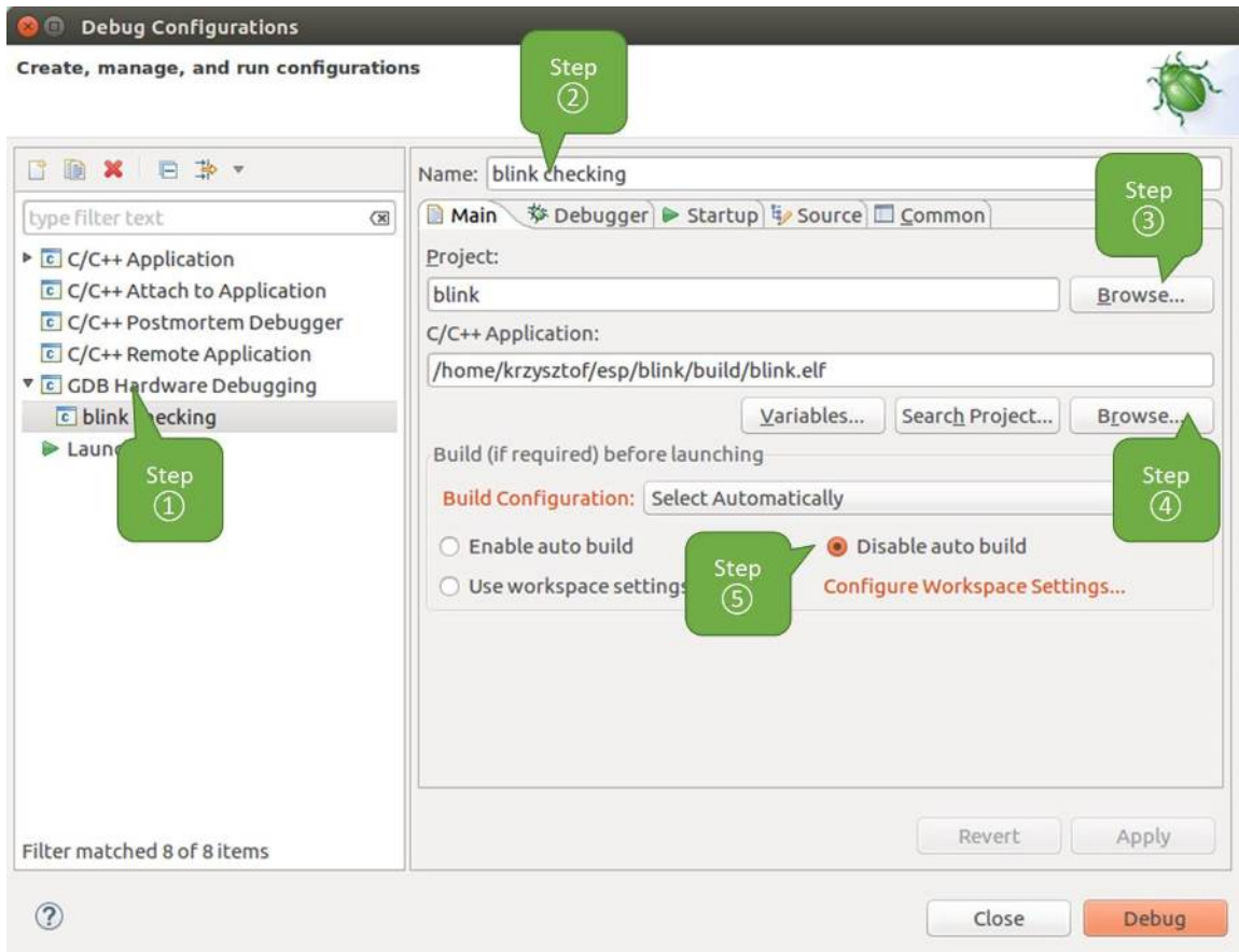
图 44: GDB 硬件调试的配置 - Main 选项卡
