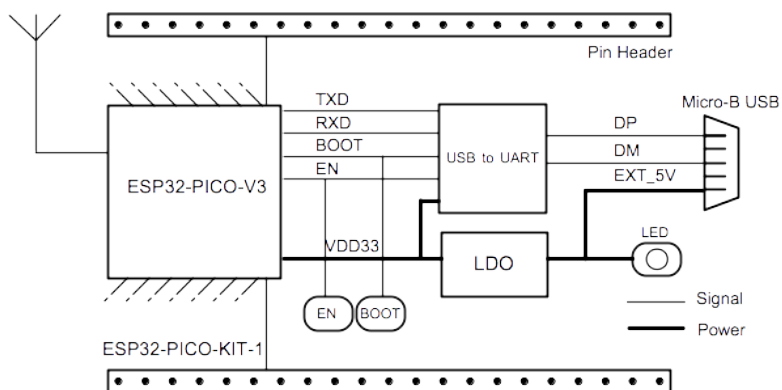
图 14: ESP32-PICO-KIT-1 功能框图 (点击放大)
