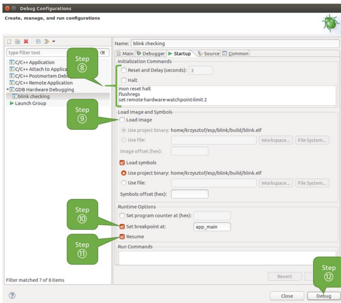
图 46: GDB 硬件调试的配置 - Startup 选项卡
