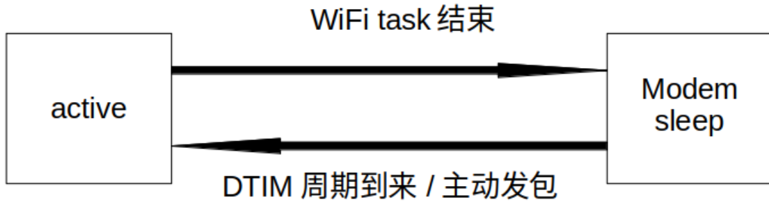
图 89: Modem sleep 工作流程图
