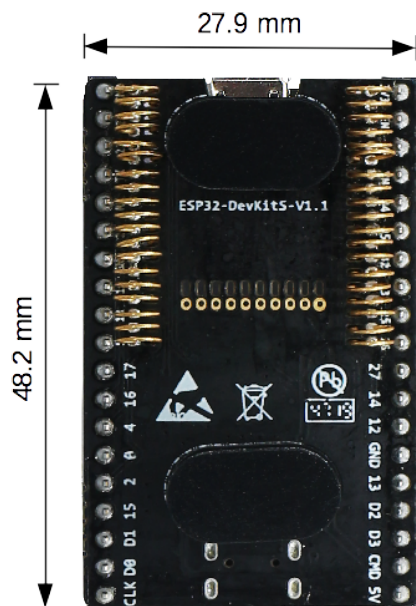
图 10: ESP32-DevKitS-R 尺寸 - 背面
