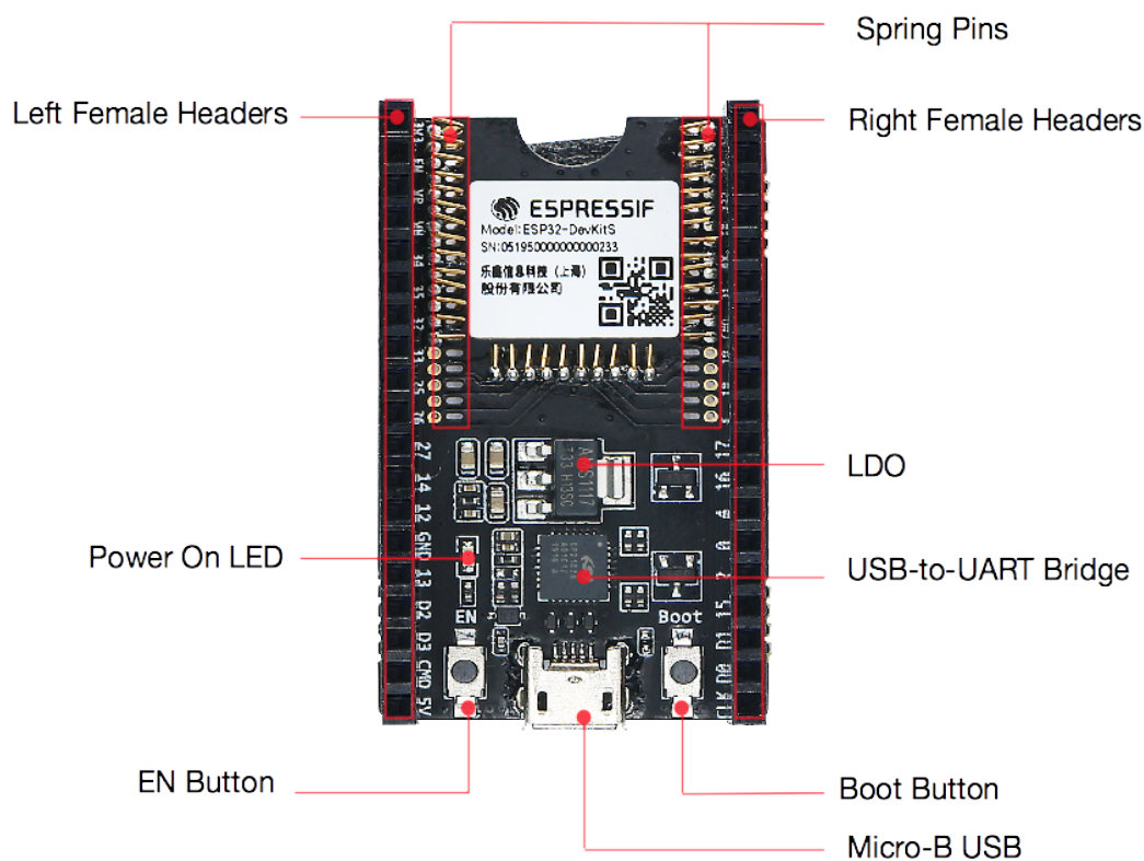
图 7: ESP32-DevKitS - 正面
