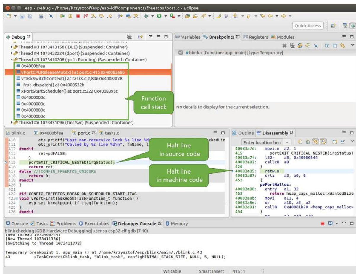
图 50: 浏览函数调用堆栈
