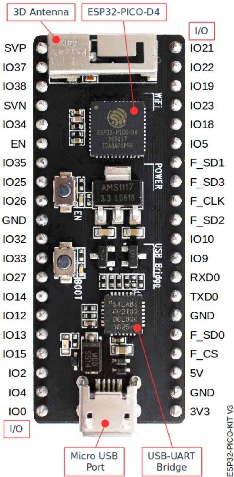
图 6: ESP32-PICO-KIT V3 开发板布局
