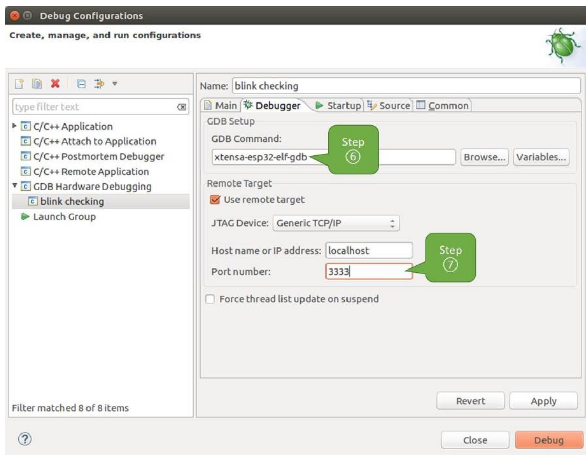
图 45: GDB 硬件调试的配置 - Debugger 选项卡
