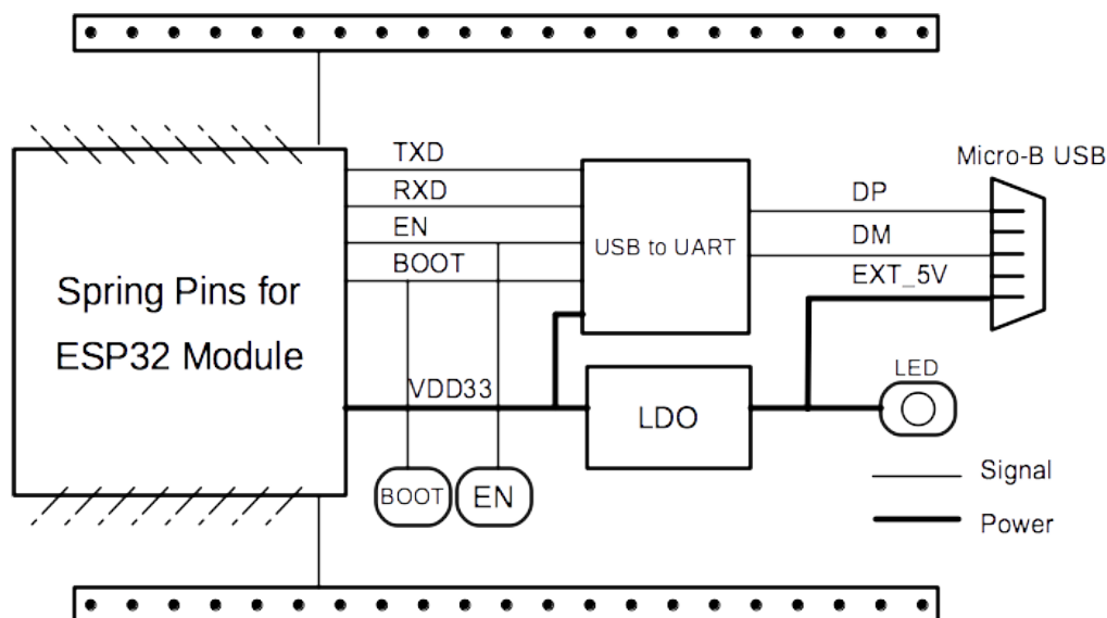
图 11: ESP32-DevKitS(-R) (点击放大)
