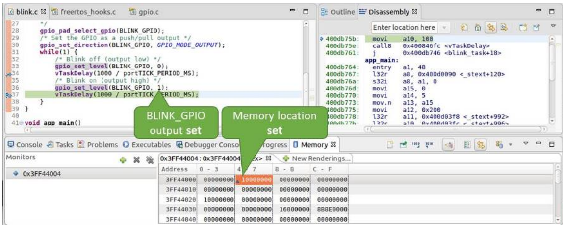
图 56: 观察内存地址 0x3FF44004 处的某个比特被置高
