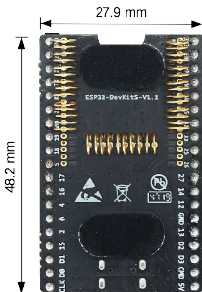
图 9: ESP32-DevKitS 尺寸 - 背面
