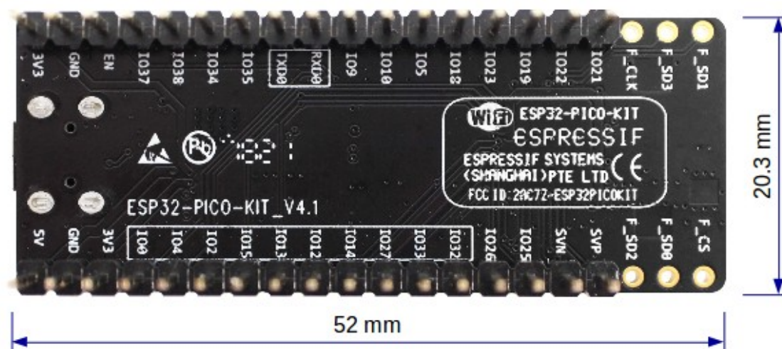
图 4: ESP32-PICO-KIT 尺寸图 -- 背面 (排针版)
