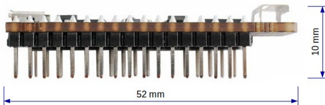
图 5: ESP32-PICO-KIT 尺寸图 -- 侧面 (排针版)
