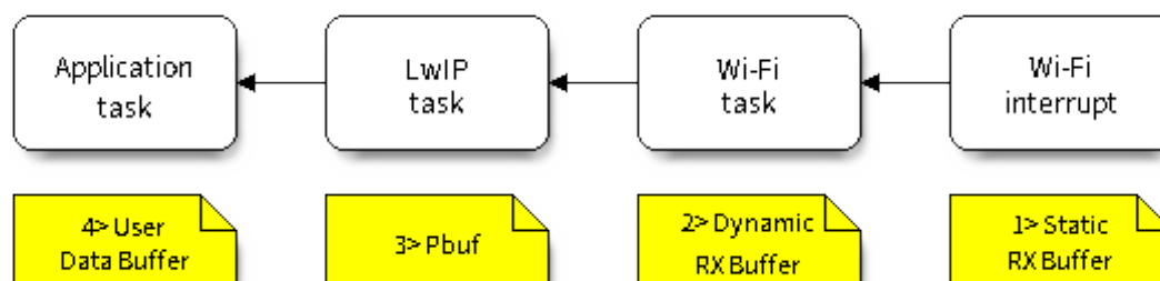
图 70: 接收数据缓冲区分配
