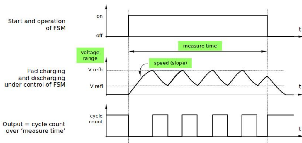
图 27: 触摸传感器 - 测量参数之间的关系
