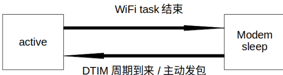
图 109: Modem sleep 工作流程图
