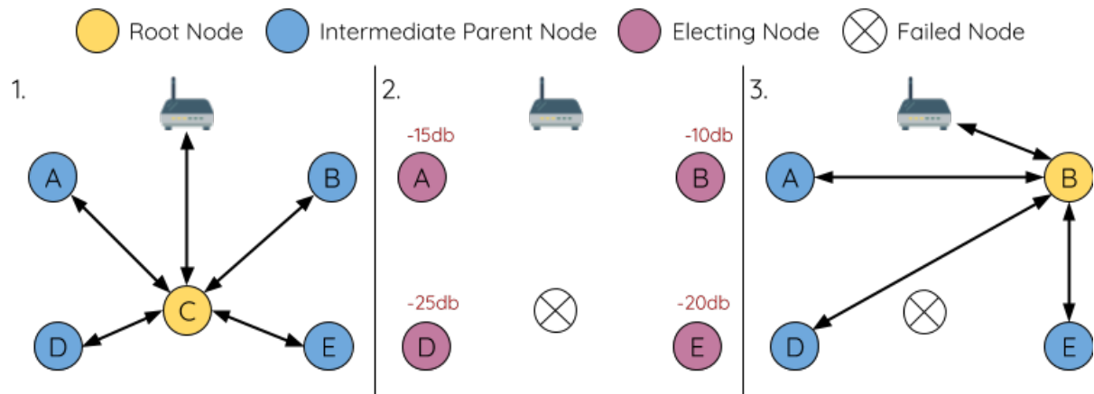
图 57: 根节点故障的自修复示意
