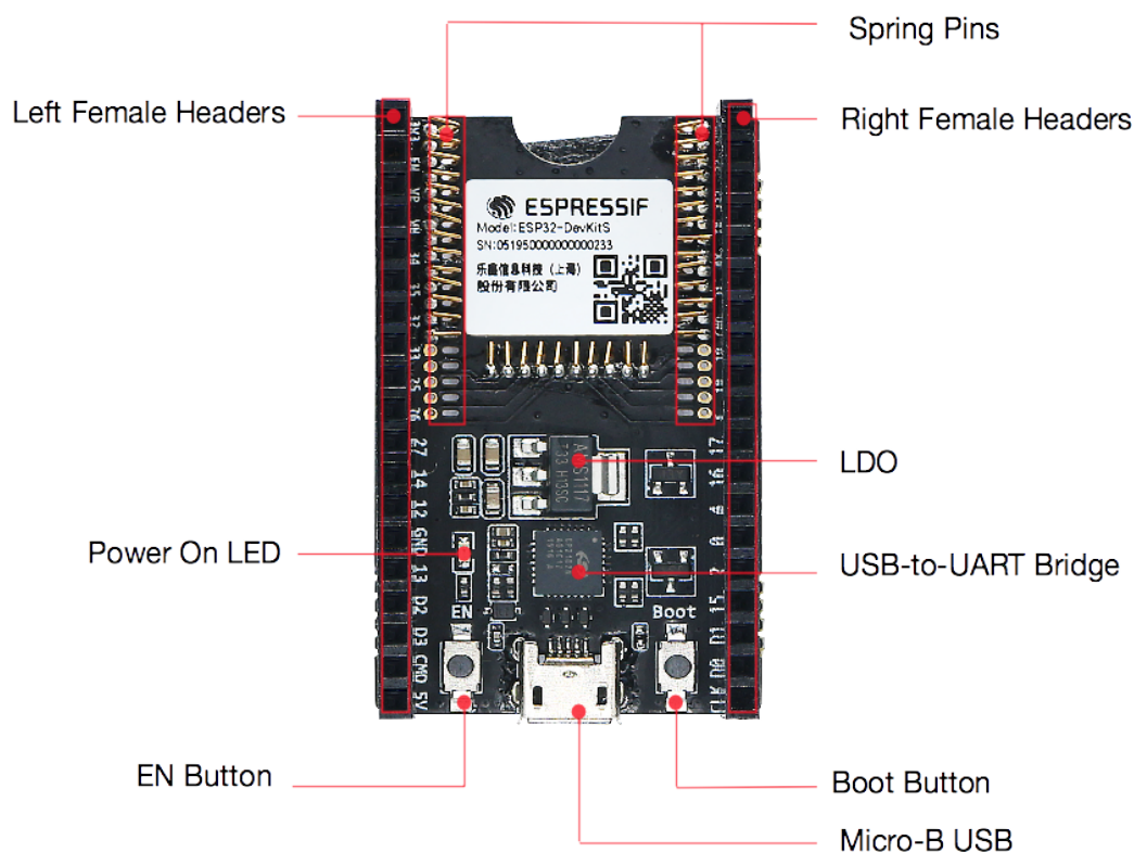
图 1: ESP32-DevKitS - 正面
