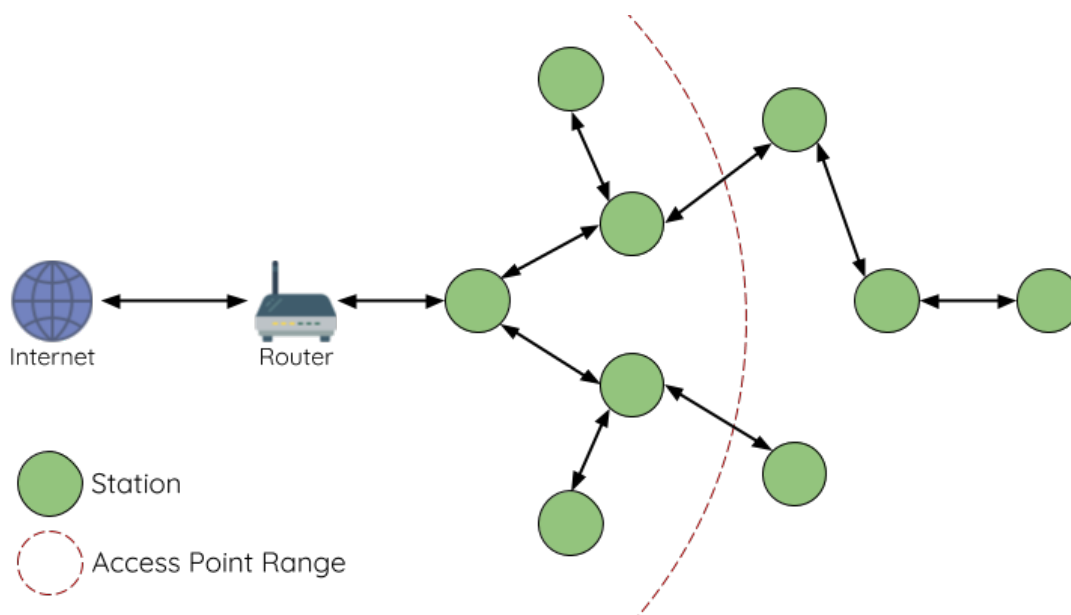
图 47: ESP-WIFI-MESH 网络架构示意图
