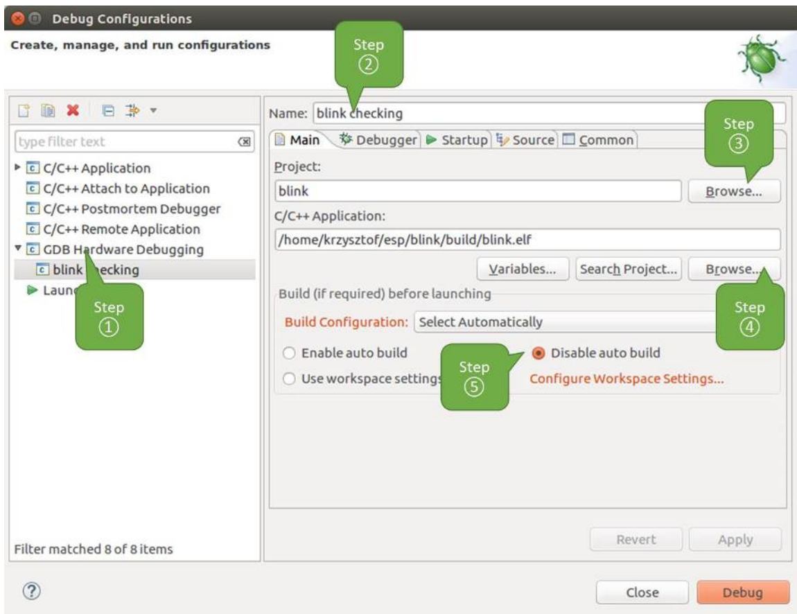
图 64: GDB 硬件调试的配置 - Main 选项卡
