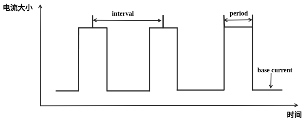
图 108: 理想情况下 Wi-Fi 场景低功耗模式电流图
