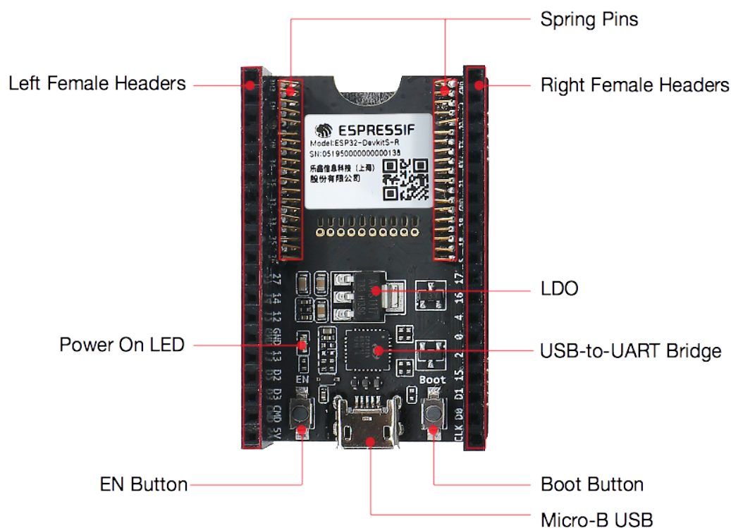
图 2: ESP32-DevKitS-R - 正面
