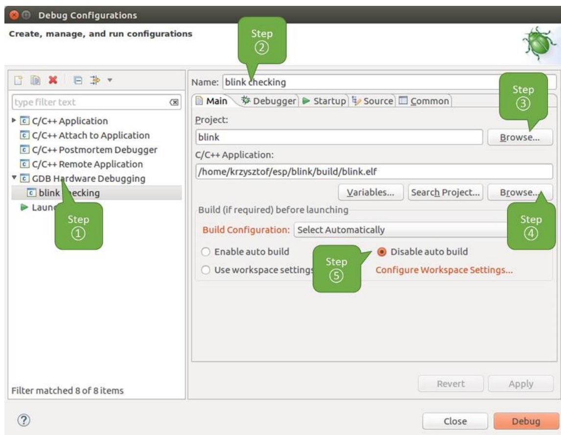
图 15: GDB 硬件调试的配置 - Main 选项卡
