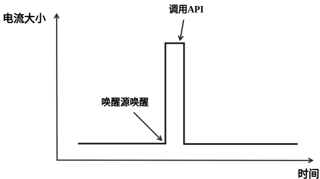
图 56: Deep-sleep 模式理想电流图
