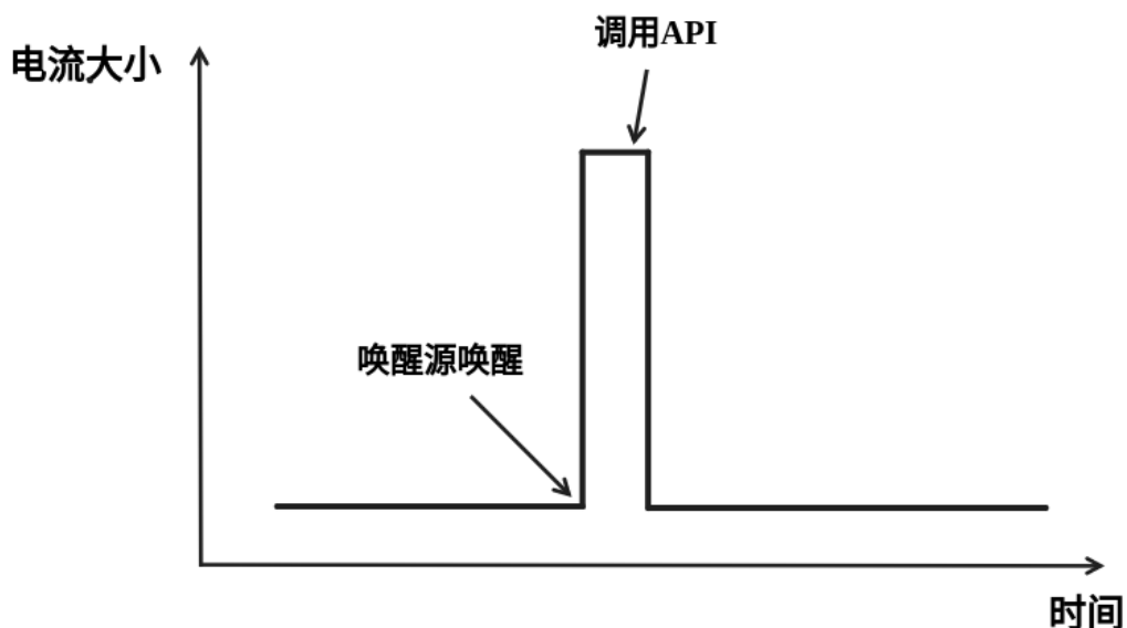
图 76: Deep-sleep 模式理想电流图
