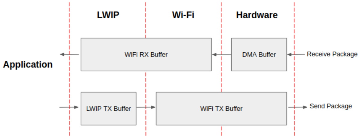
图 59: ESP32-C2 数据路径
