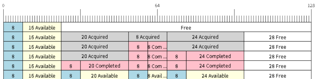
图 16: 在不可分割环形 buffer 中 SendAcquire/SendComplete 数据项
