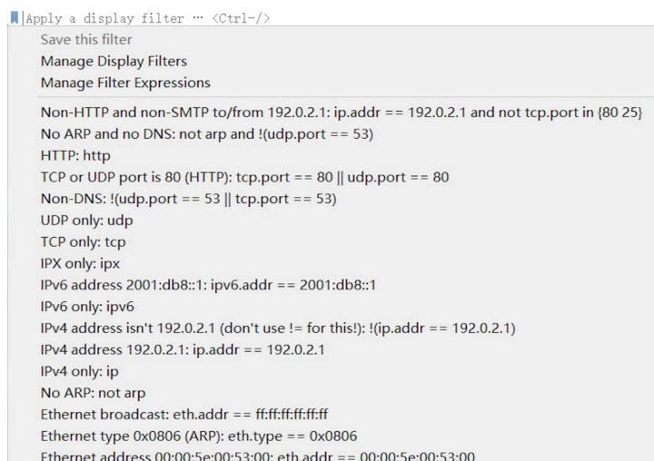
图 64: Display Filter 对话框
