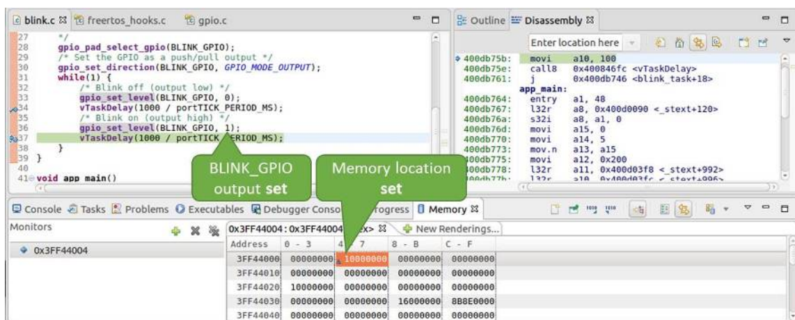
图 47: 观察内存地址 0x3FF44004 处的某个比特被置高
