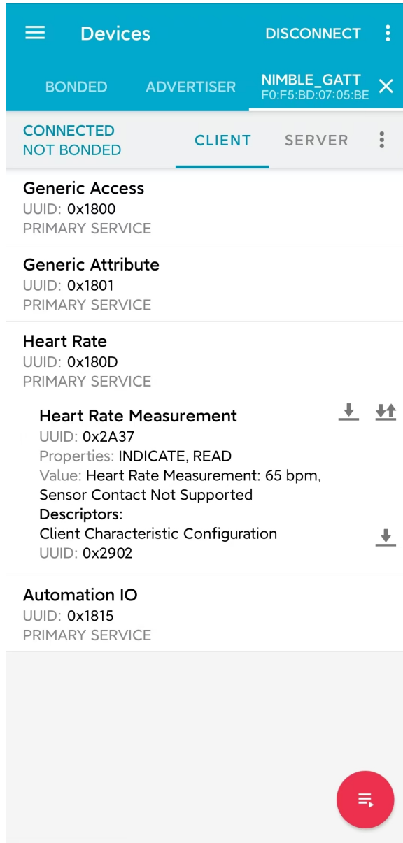
图 12: 对心率特征数据进行读访问
