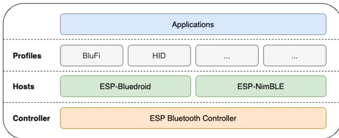
图 2: ESP32-C2 蓝牙协议栈架构
