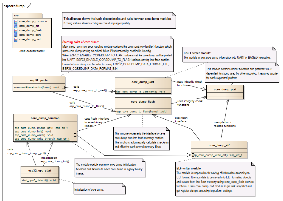
图 29: 核心转储实现
