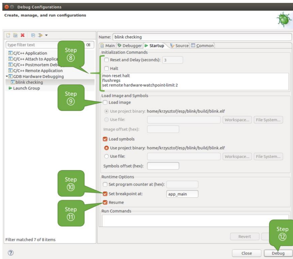
图 37: GDB 硬件调试的配置 - Startup 选项卡
