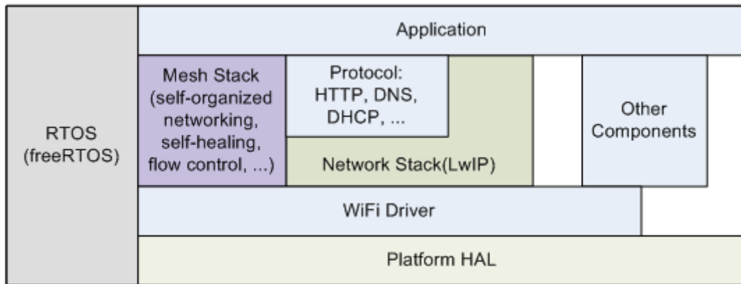
图 2: ESP-WIFI-MESH 软件栈
