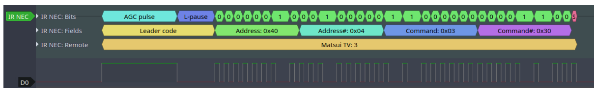
图 25: 红外 NEC 帧
