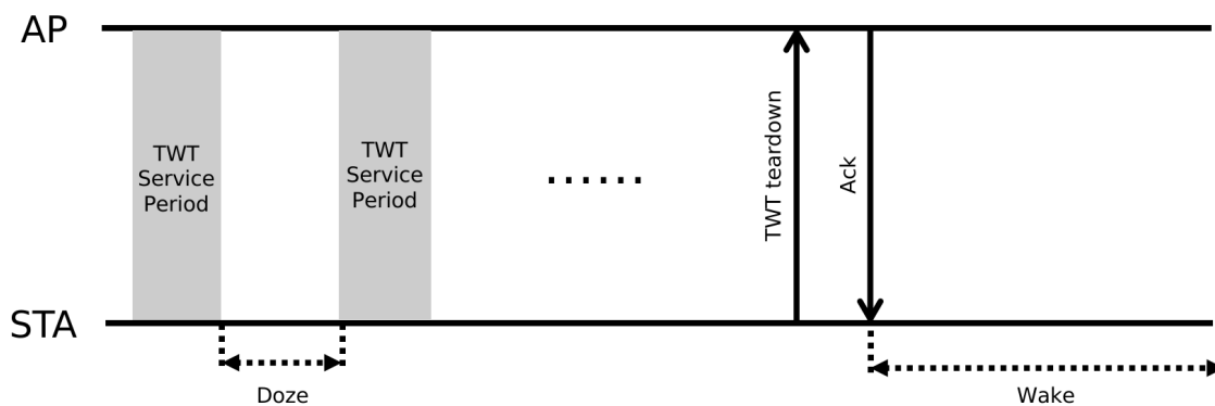
图 115: Individual TWT 协商终止过程示例
