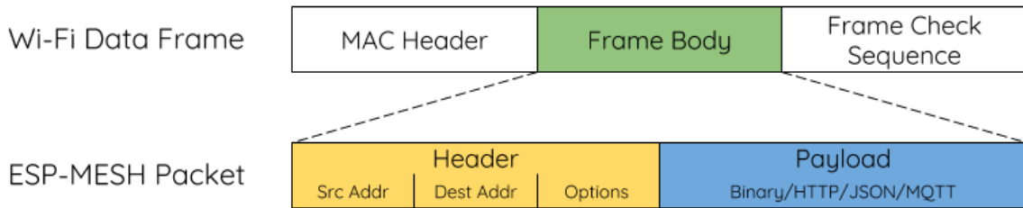
图 58: ESP-WIFI-MESH 数据包
